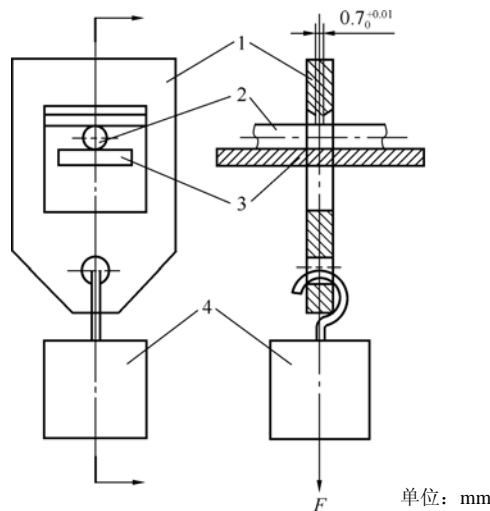
1——试验构架；2——样品；3——支架；4——砝码。
