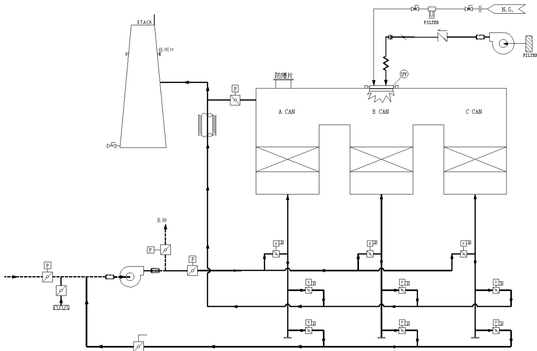
图 A.2 不通过排放口排放的 RTO 废气旁路示意图
