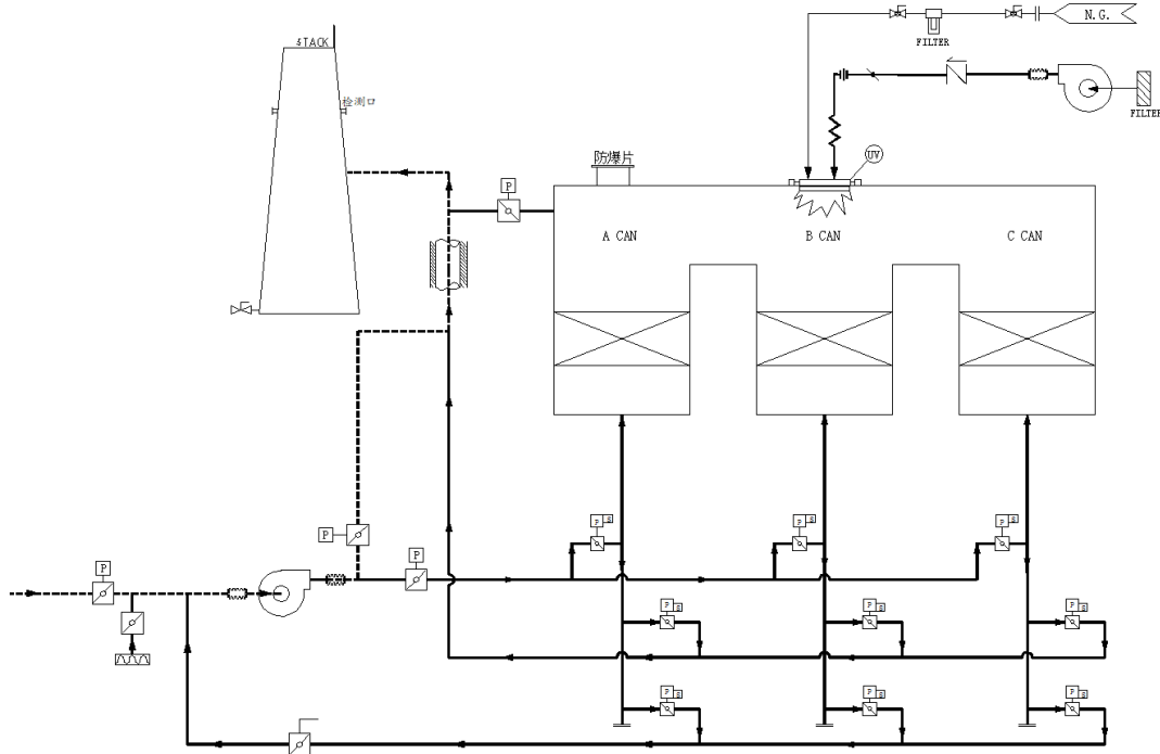
图 A.1 通过排放口排放的 RTO 废气旁路示意图
