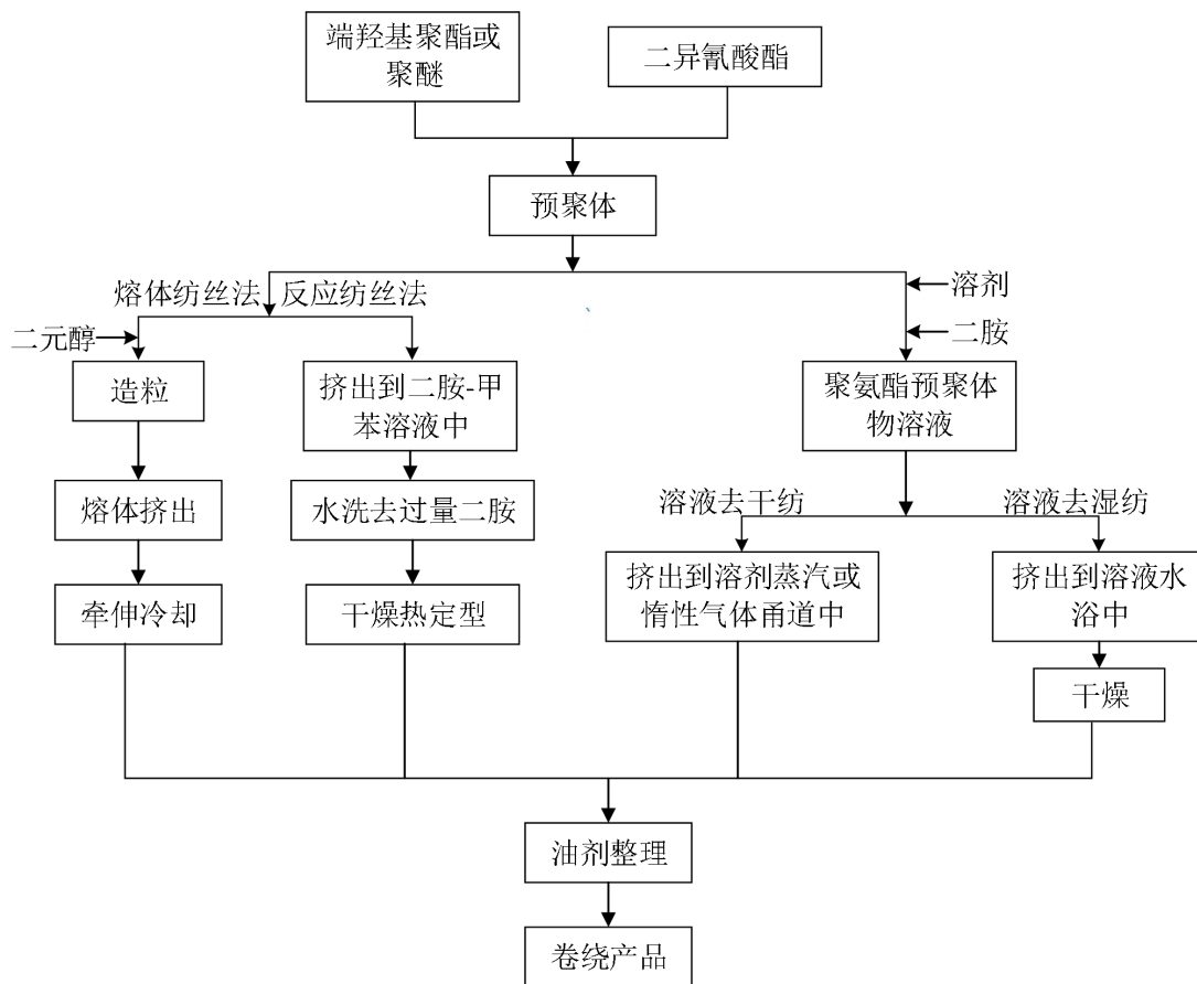
图 A.2 氨纶工艺流程
