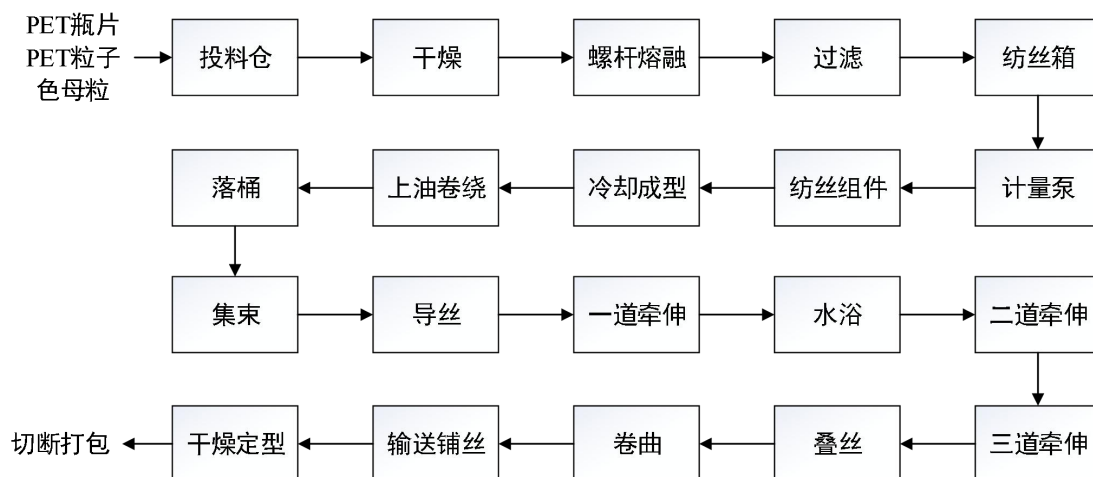
图 A.3 再生涤纶工艺流程
