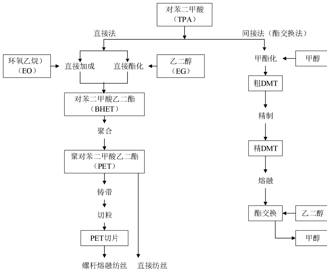
图 A.1 涤纶工艺流程
