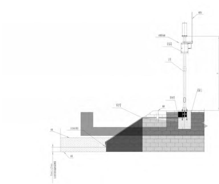
图 9-11 压力水位计立杆式安装示意图
