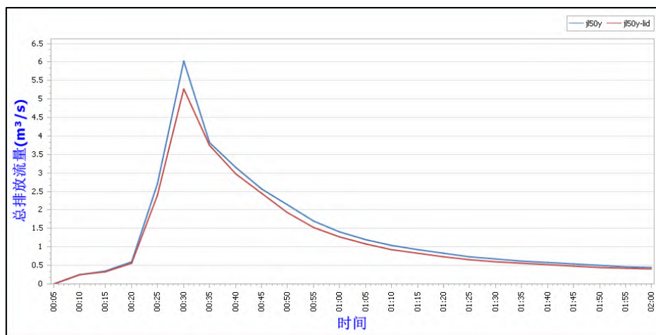
图 10-30 50 年一遇低影响开发前后总排放流量对比分析
