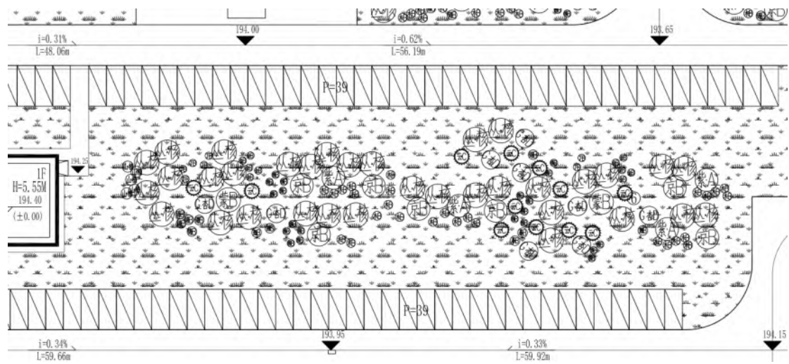
图 10-15 绿地类海绵城市设施植物种植设计图
