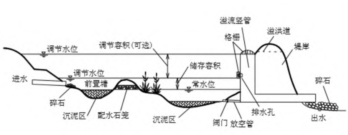
图 8-7 湿塘典型构造示意图
