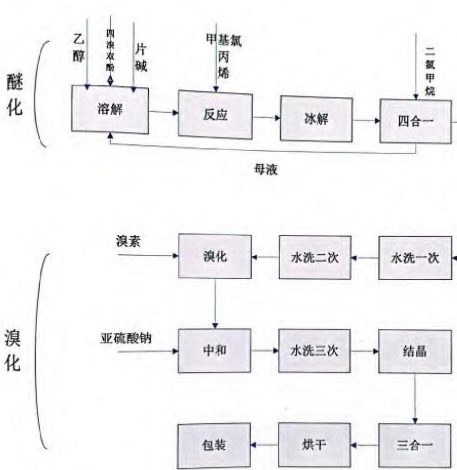
甲基八溴醚工艺流程图
