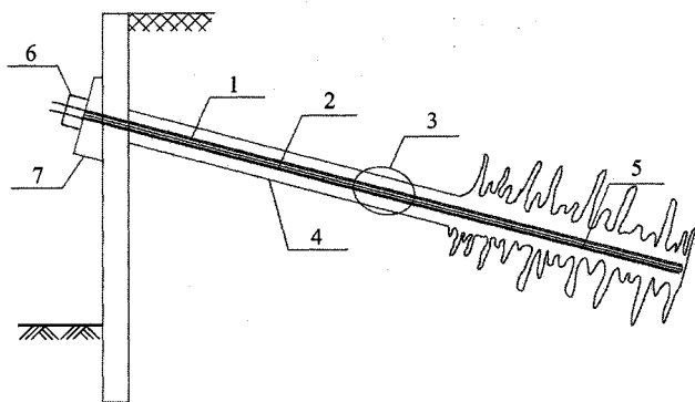
图 4.2.6 可重复高压灌浆型锚杆结构简图
