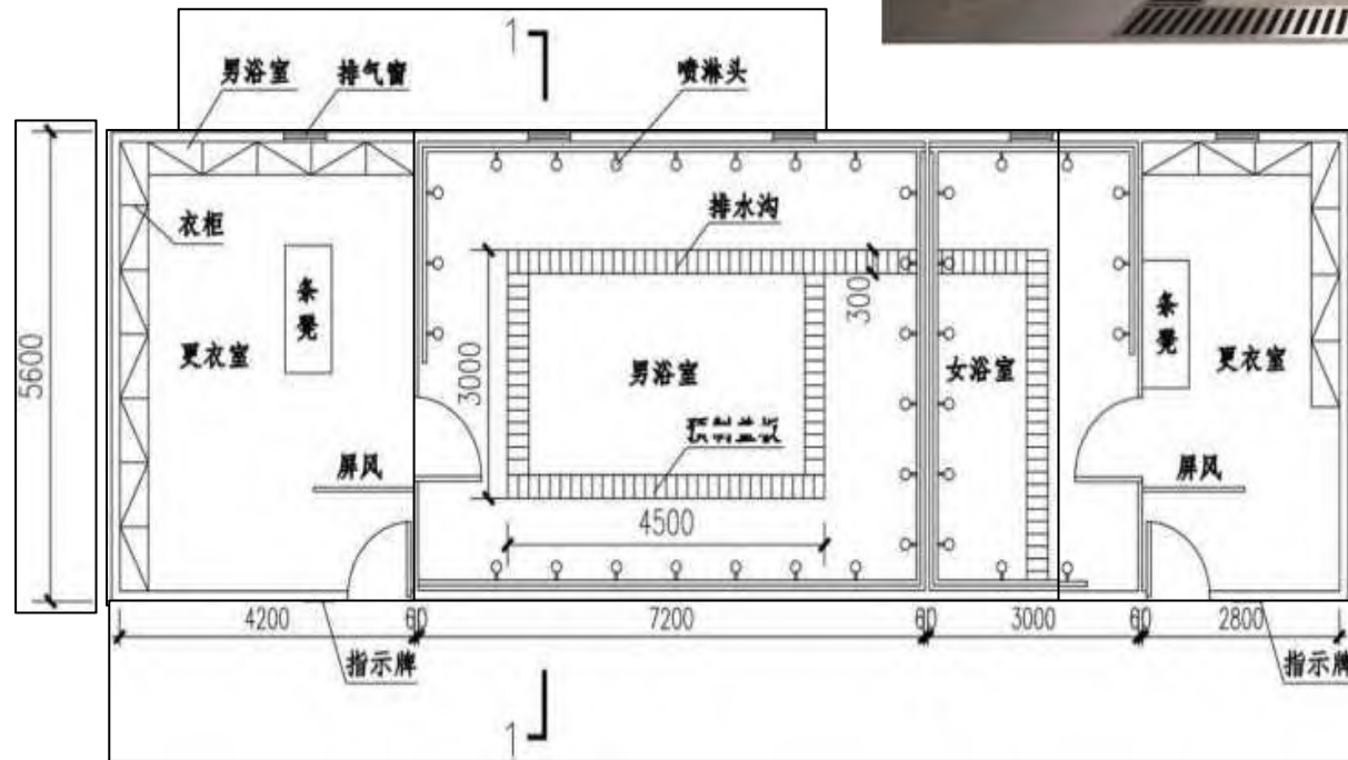
浴室平面图
