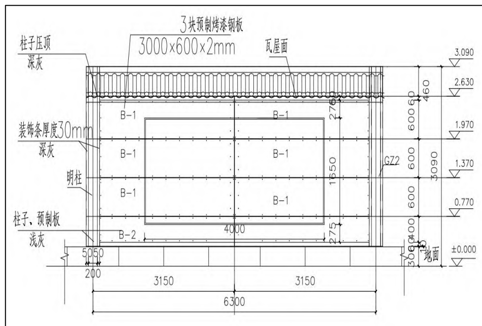
传统风格钢结构装配式围挡立面图
