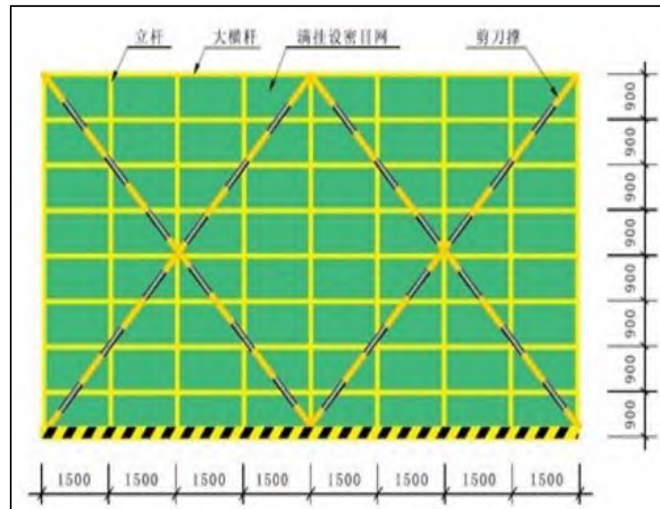
脚手架剪刀撑交叉点设置示例图
