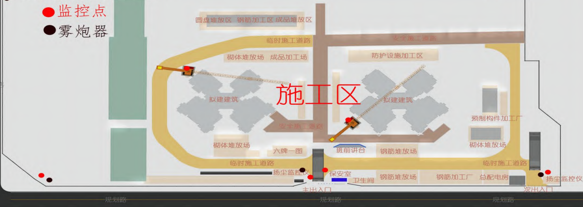
施工总平面布置图示例
