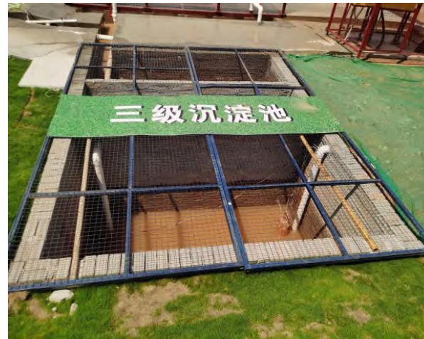
三级沉淀池示例图
