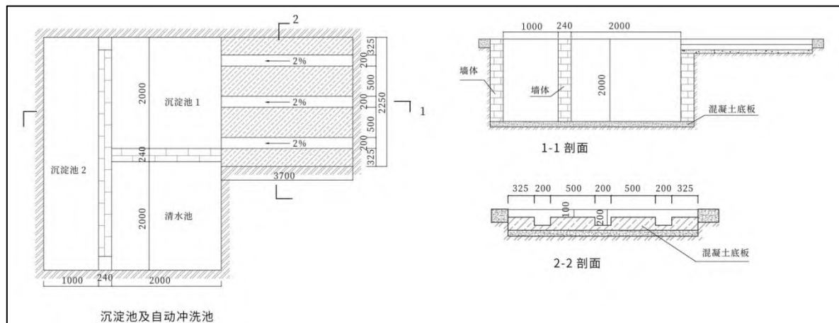
冲洗设施及沉淀池施工图
