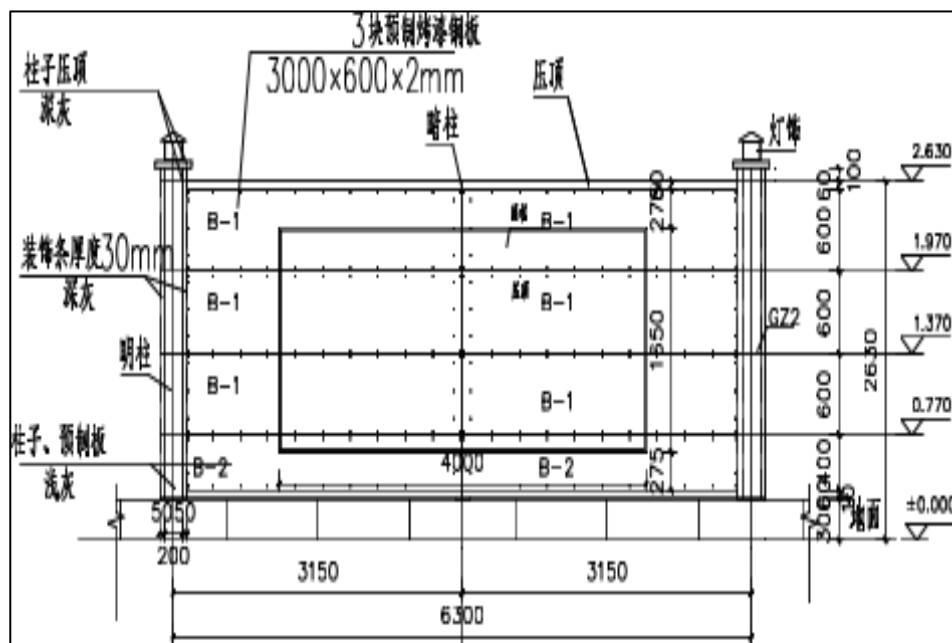
现代风格钢结构装配式围挡示意图
