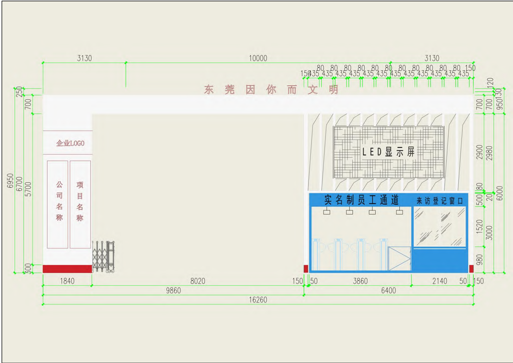
主入口大门正面参考尺寸图（单位：mm）
