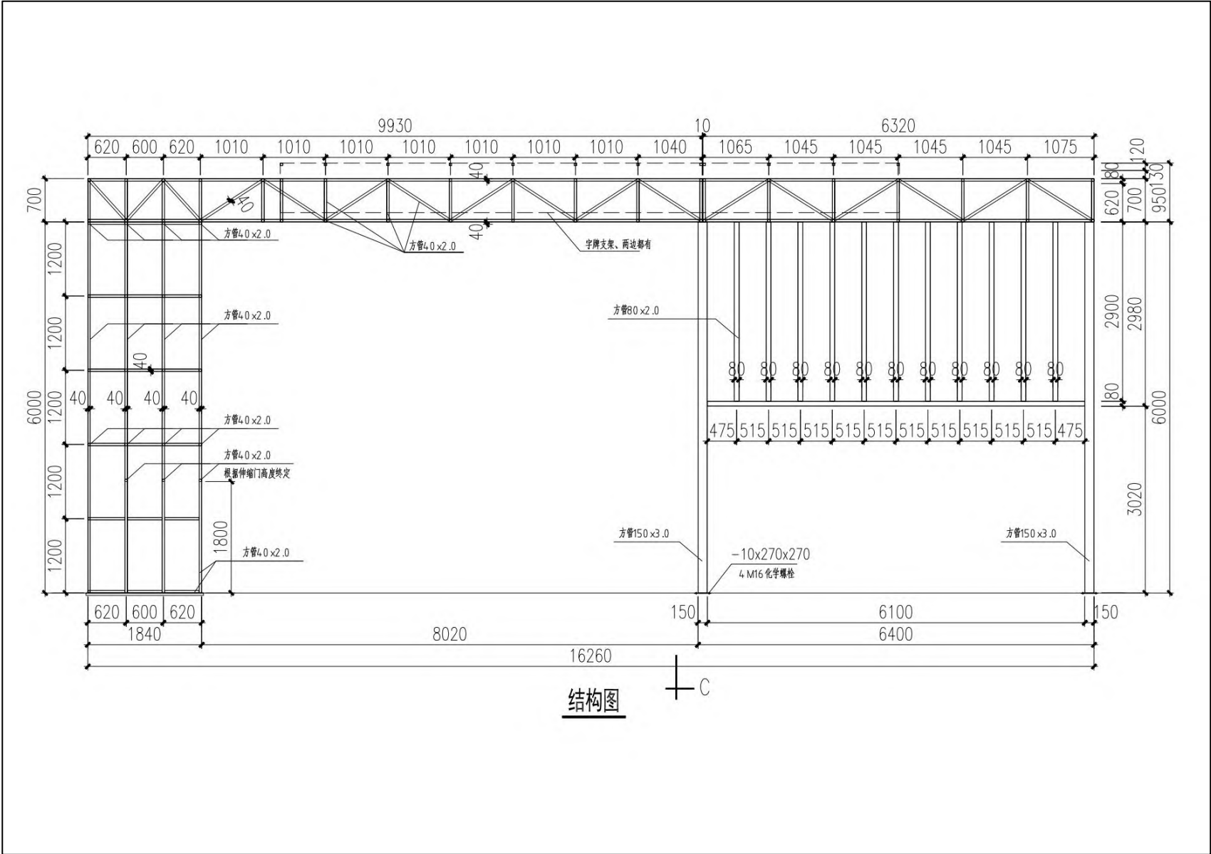
主出入口大门结构参考尺寸图（单位：mm）
