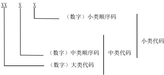
图2 代码结构图
