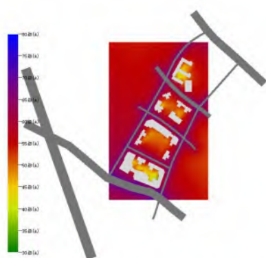
项目1.5m高度处声压级平面分布图（昼间）
