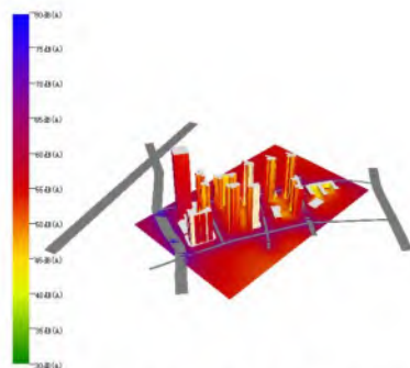
建筑立面噪声级分布图（昼间）
