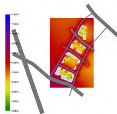
项目1.5m高度处声压级平面分布图（夜间）
