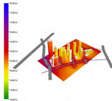
建筑立面噪声级分布图（夜间）
