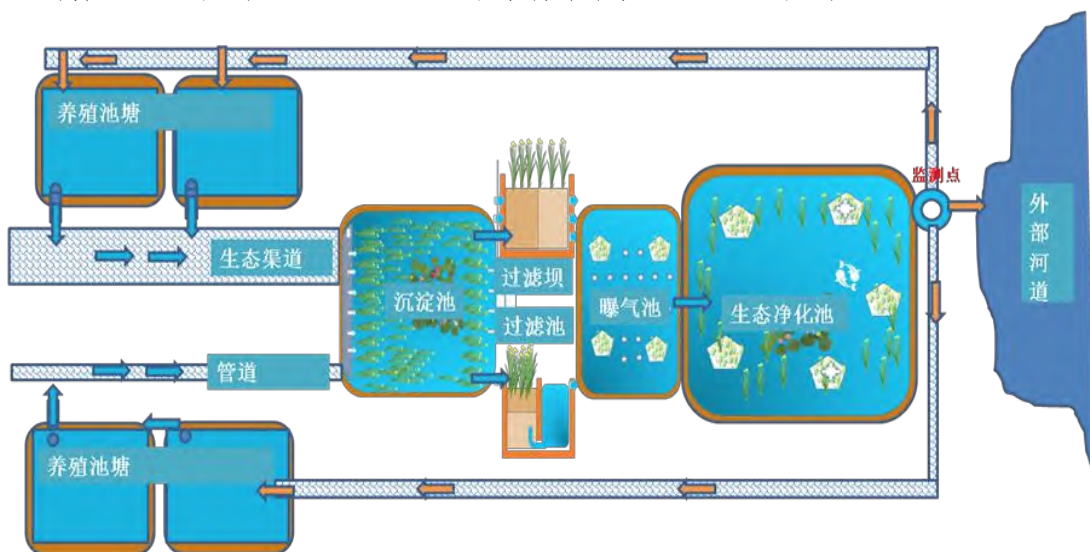
图 2 池塘养殖水生态治理标准处理工艺流程图
