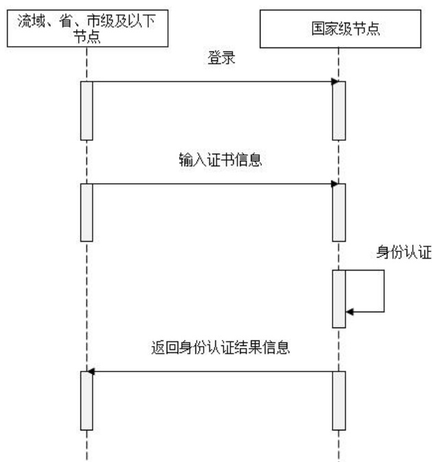
图 2 身份认证流程图
