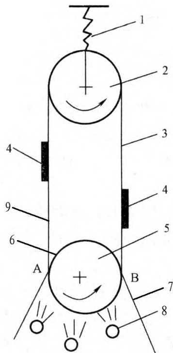
图3-9 圆形曝光
