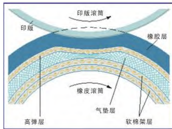
气垫橡皮布
