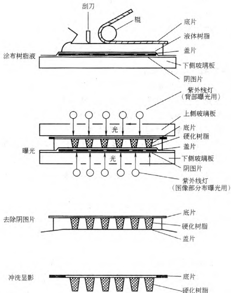
图 3-10 液体感光树脂柔性版制作工艺流程
