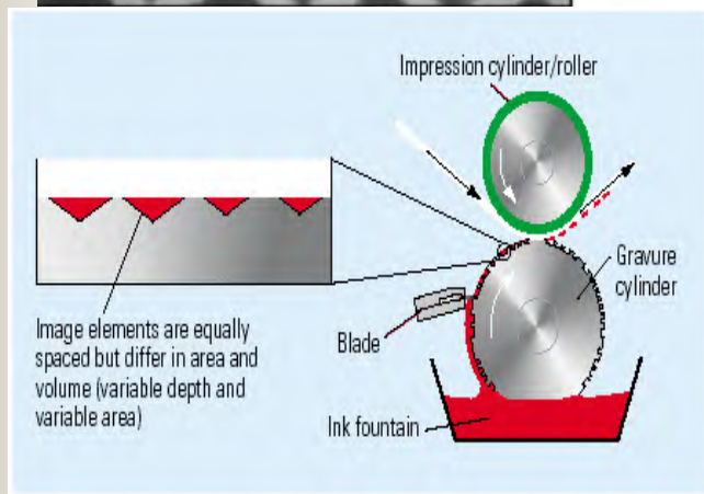
凹版网墙
