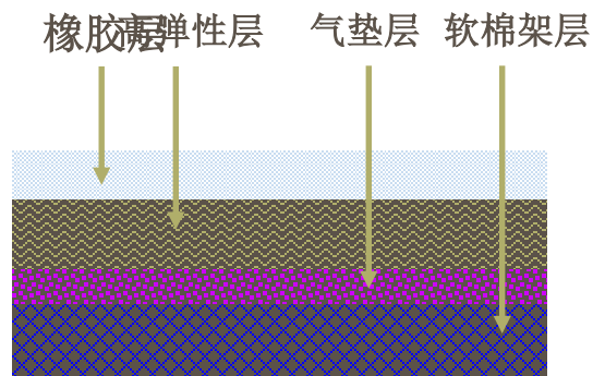
气垫橡皮布
