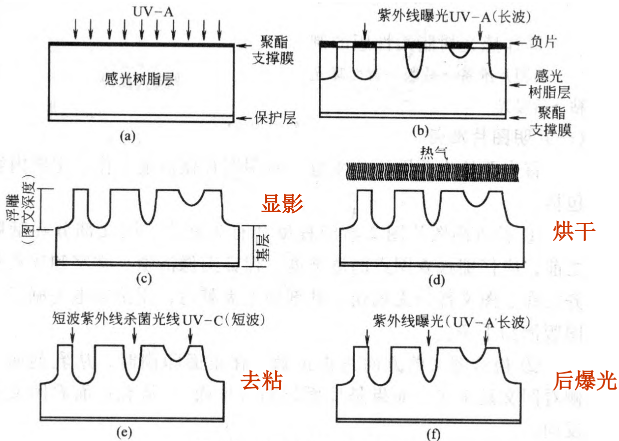
图 3-8 赛丽版制作工艺
