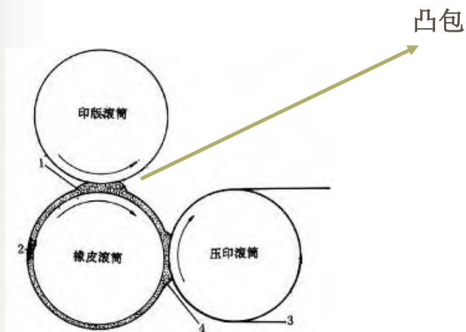
普通橡皮布
