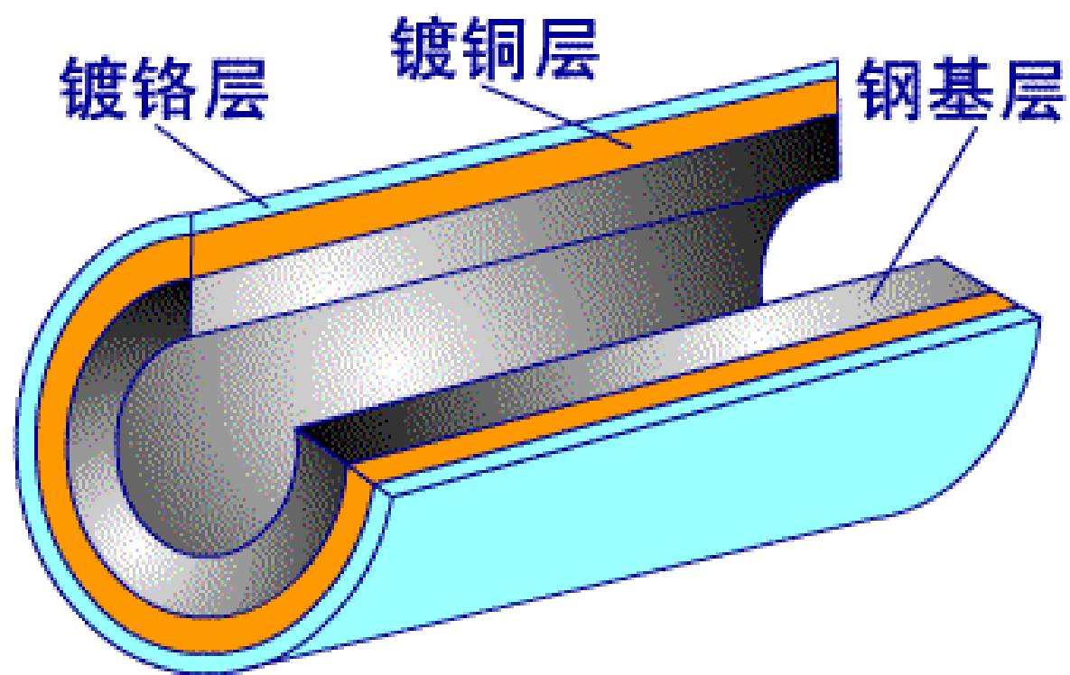
凹版滚筒（版辊）
