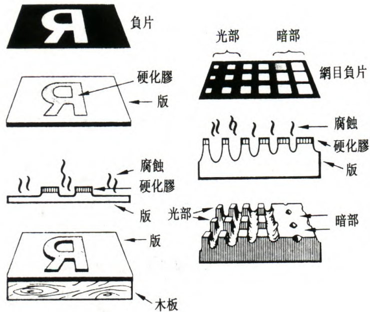
照相凸版
