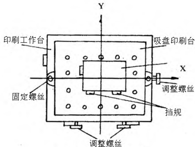
半自动丝网印刷机定规矩
