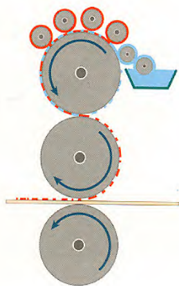
平版印刷原理圖解
