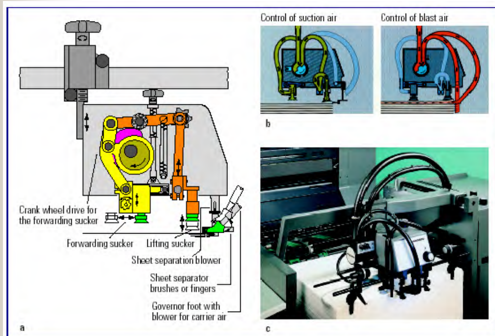
给纸机构的飞达
