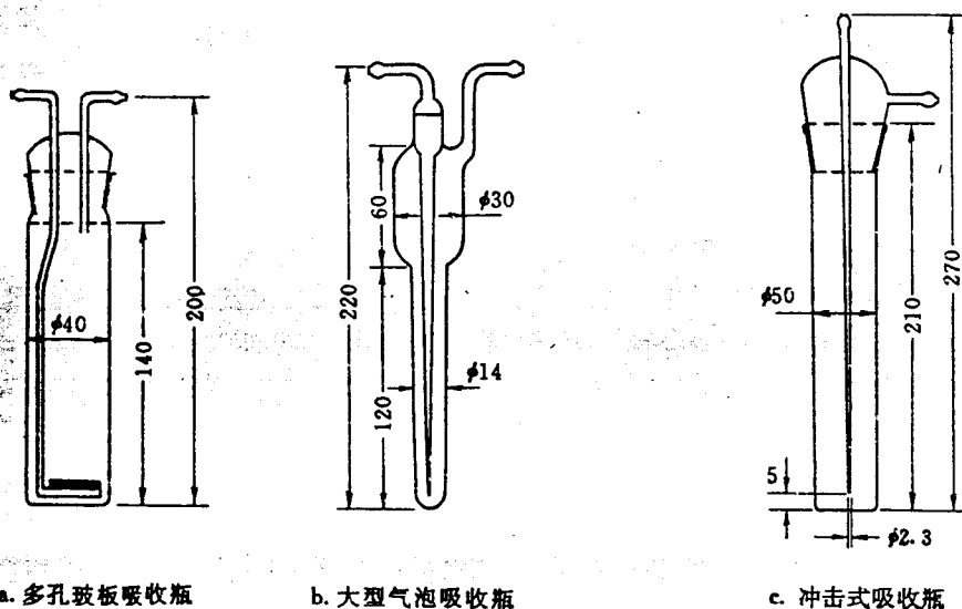
图 34 常用的几种吸收瓶
