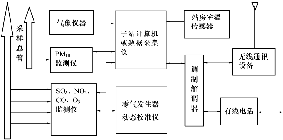
图 4-5 监测子站仪器设备配置示意图
