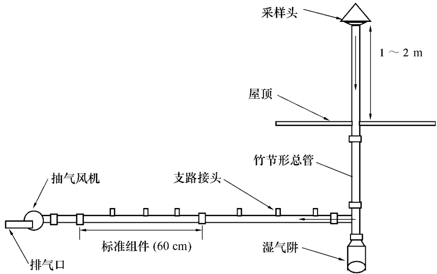
图 4-3 竹节式多路支管系统 (1)
