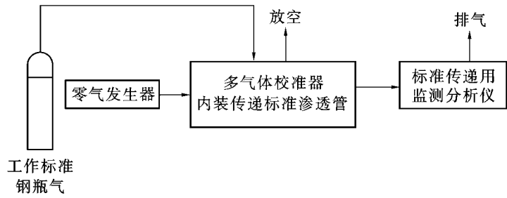
图 C.7 渗透管传递图
