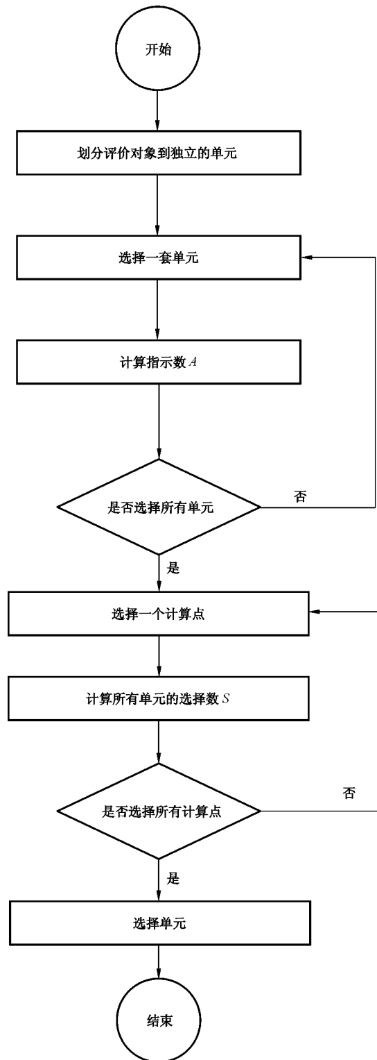
图 B.1 设备选择数法流程示意图
