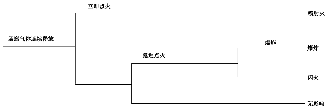
图 F.2 易燃气体连续释放事件树
