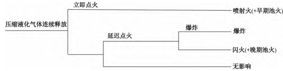
图 G.4 压缩液化气体连续释放事件树
