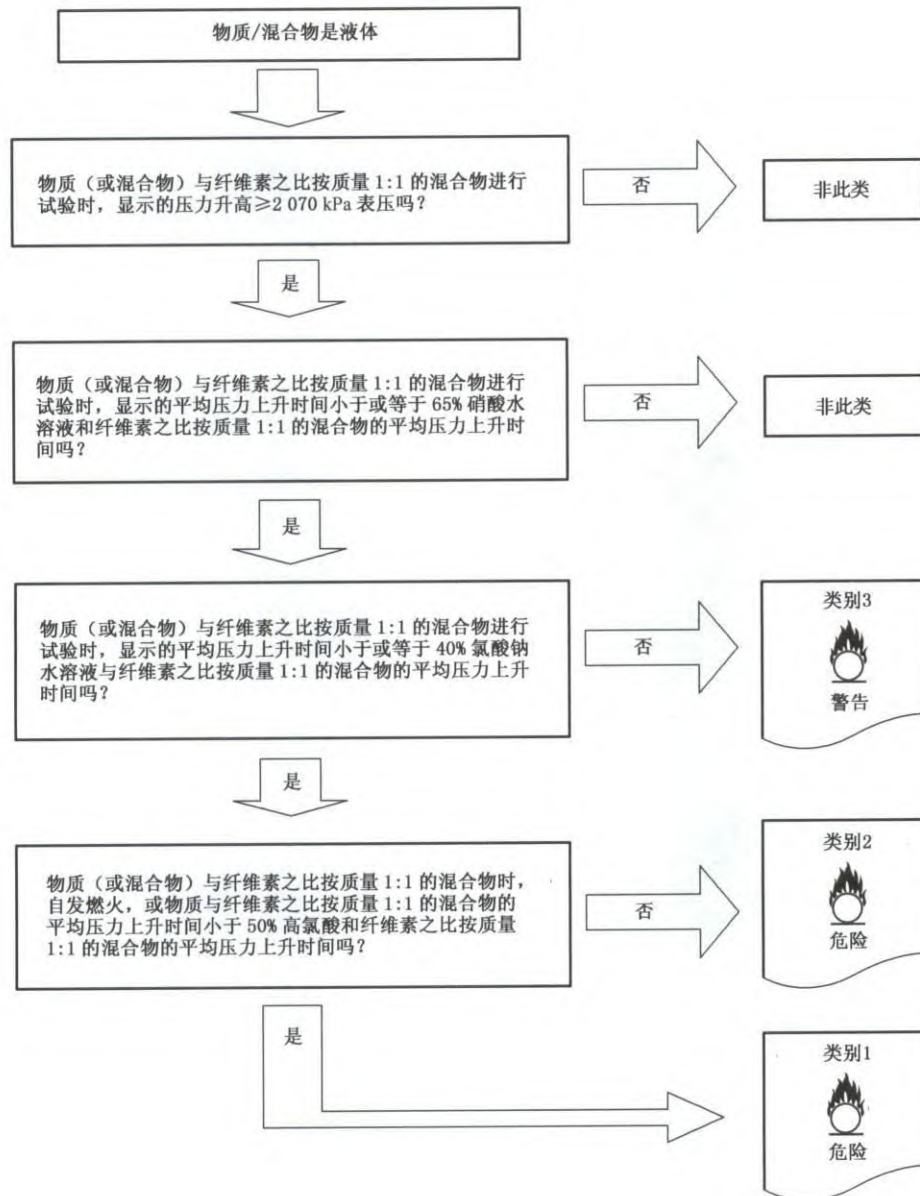
图 A.1 氧化性液体判定逻辑
