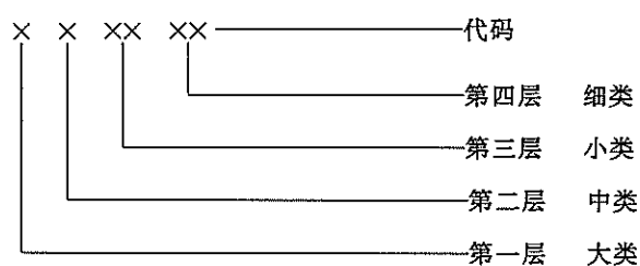
图 1 代码结构
