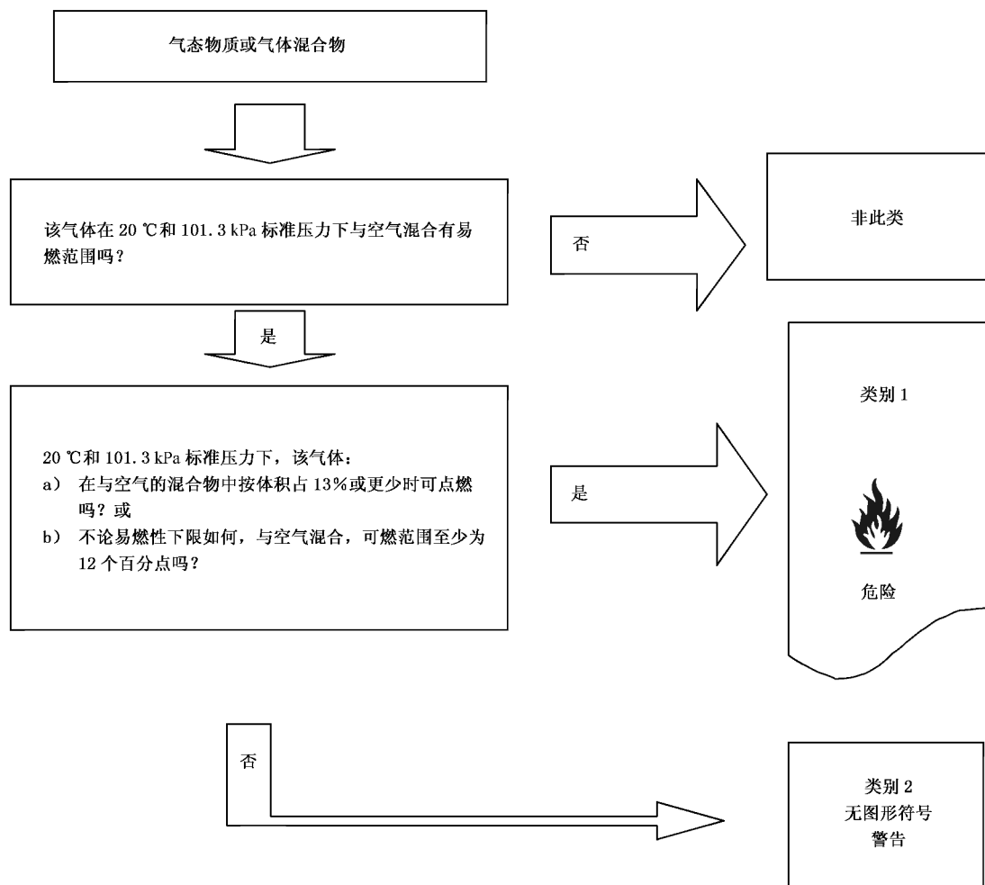
图 A.1 易燃气体的判定逻辑
