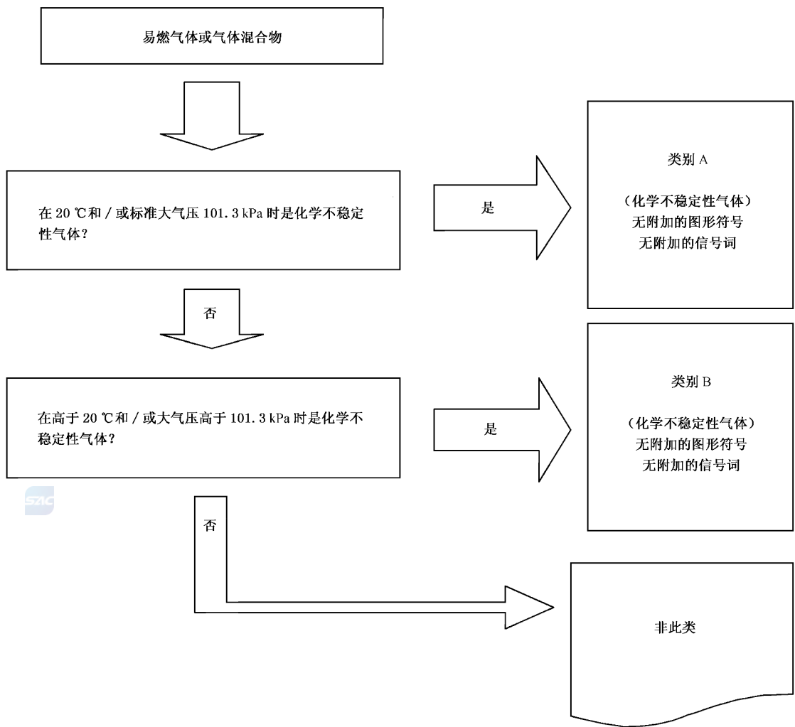
图 A.2 化学不稳定性气体的判定逻辑
