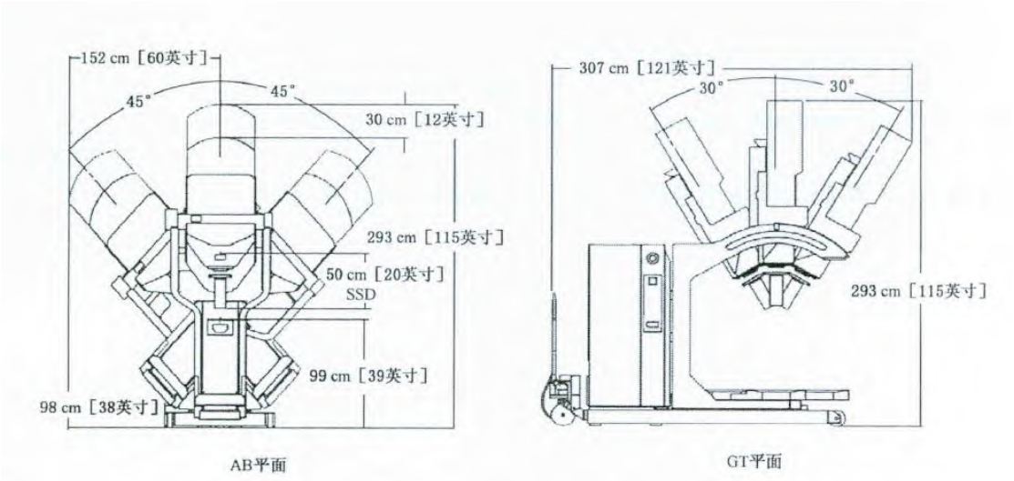
图C.1 移动加速器倾角范围示意图
