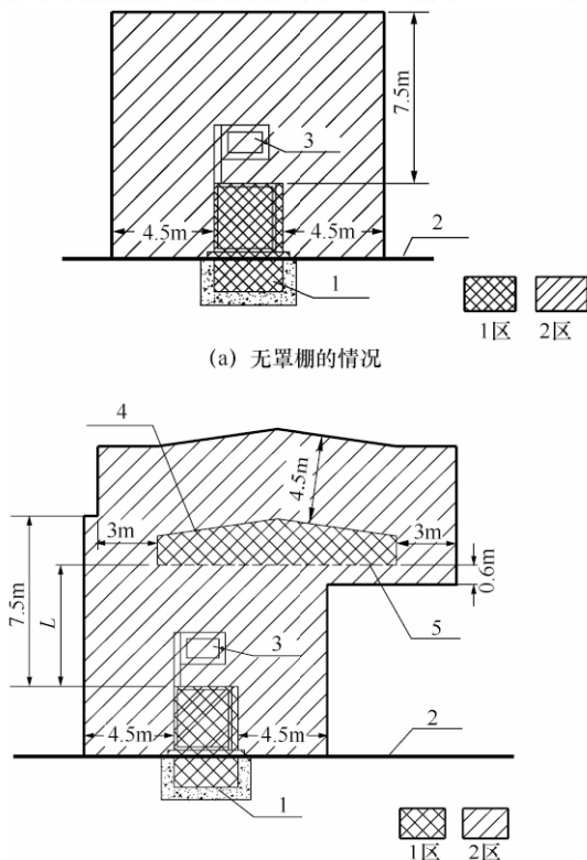
图 A.0.6 压缩天然气加气柱（装置）、卸气柱（装置）的爆炸危险区域等级和范围的划分 1—坑或沟；2—地坪；3—计量显示装置；4—罩棚顶； 5—罩棚封闭空间底部
