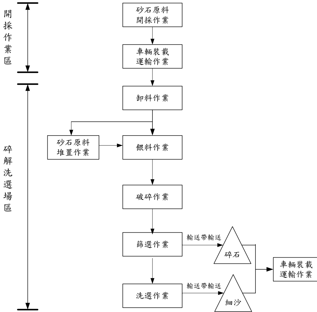
圖2-1 砂石採集處理作業流程圖
