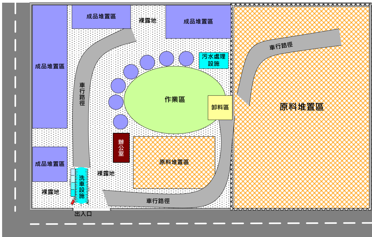
圖4.1 大型砂石場案例場區配置圖
