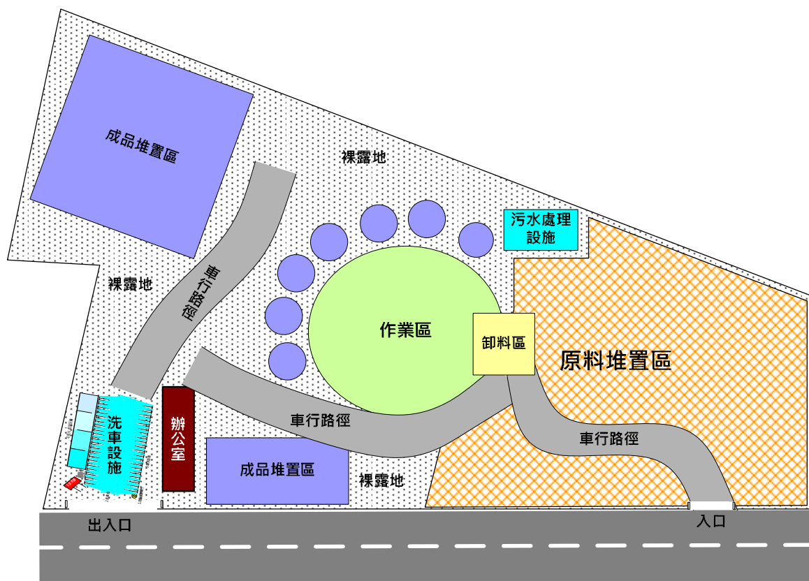
圖4.2 中型砂石場案例場區配置圖
