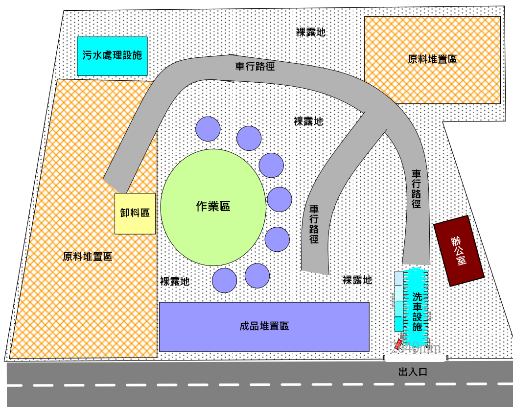
圖4.3 小型砂石場案例場區配置圖
