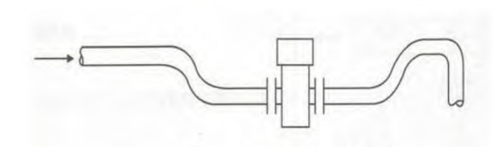
敞口排放，流量计安装要求
