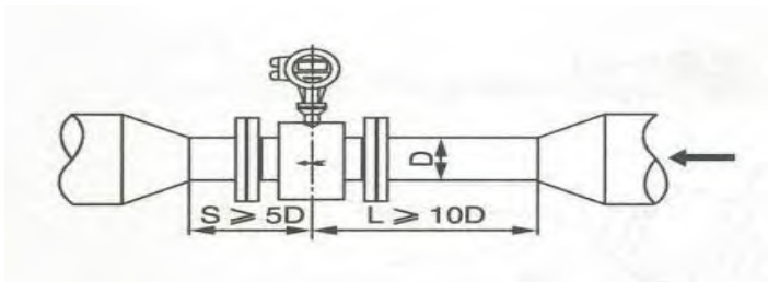
图 c 扩口管前、后直管段长度要求
