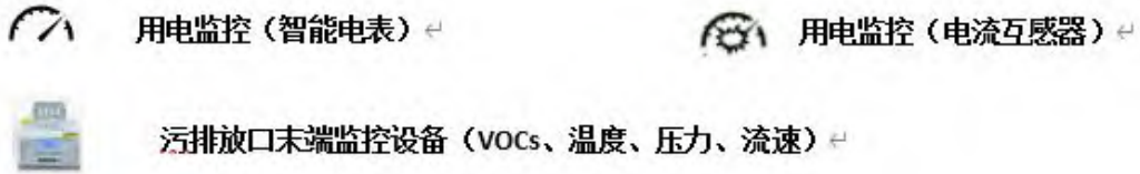
图5.6.2 东莞市涉VOCs排放企业过程、末端自动监控环节示意图
