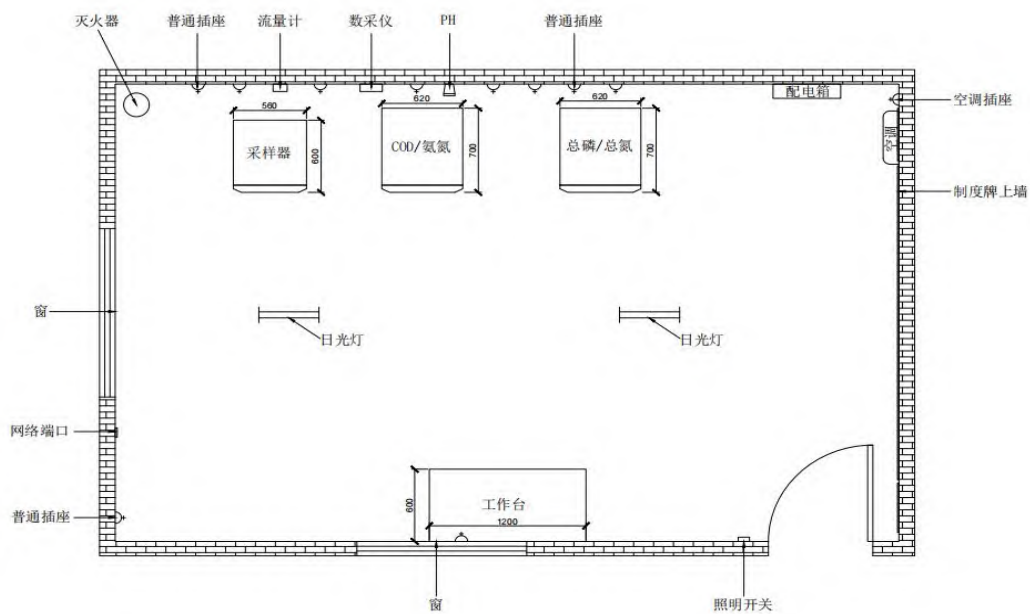
图 8.12.1 在线监控站房布局示意图
