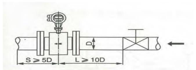
图 d 阀门下游前、后直管段长度要求
