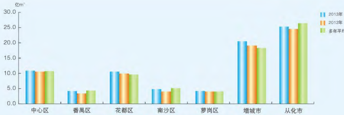
各行政区2013年地表水资源量与2012年、多年平均比较图
