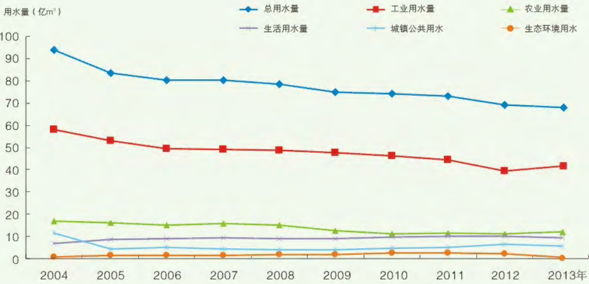
2004~2013年各类用水量变化趋势图
