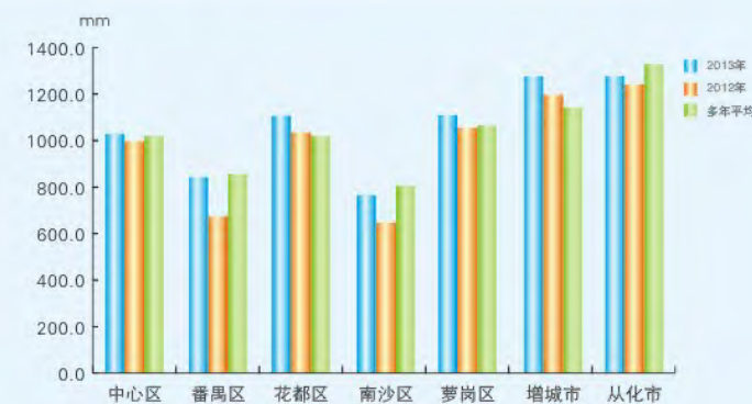
各行政区2013年径流深与2012年、多年平均比较图
