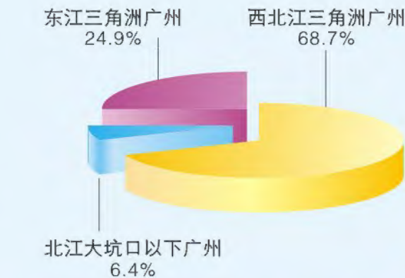
2013年各水资源分区地下水资源量对比图
