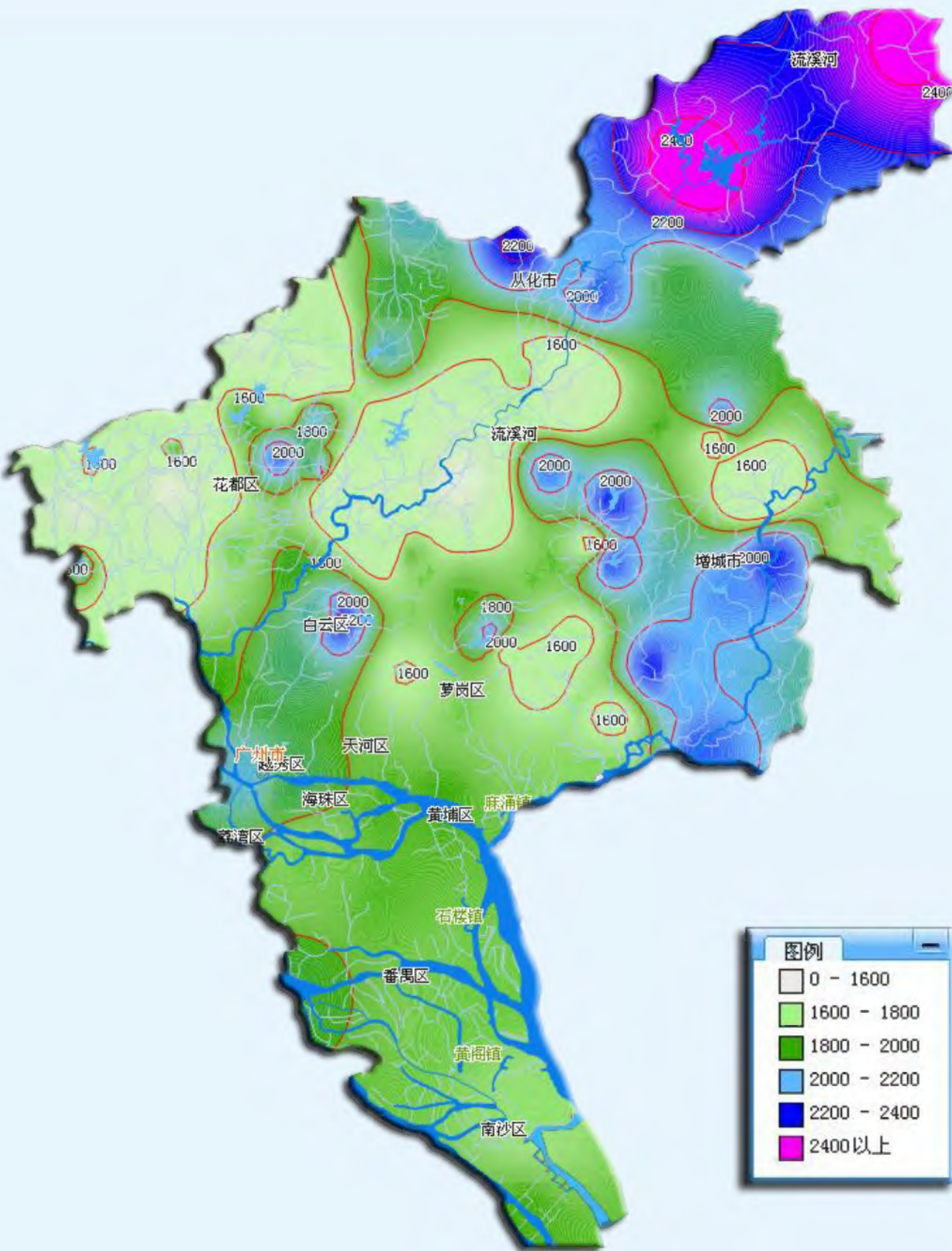
2013年广州市降雨量等值线图 (单位: mm)
