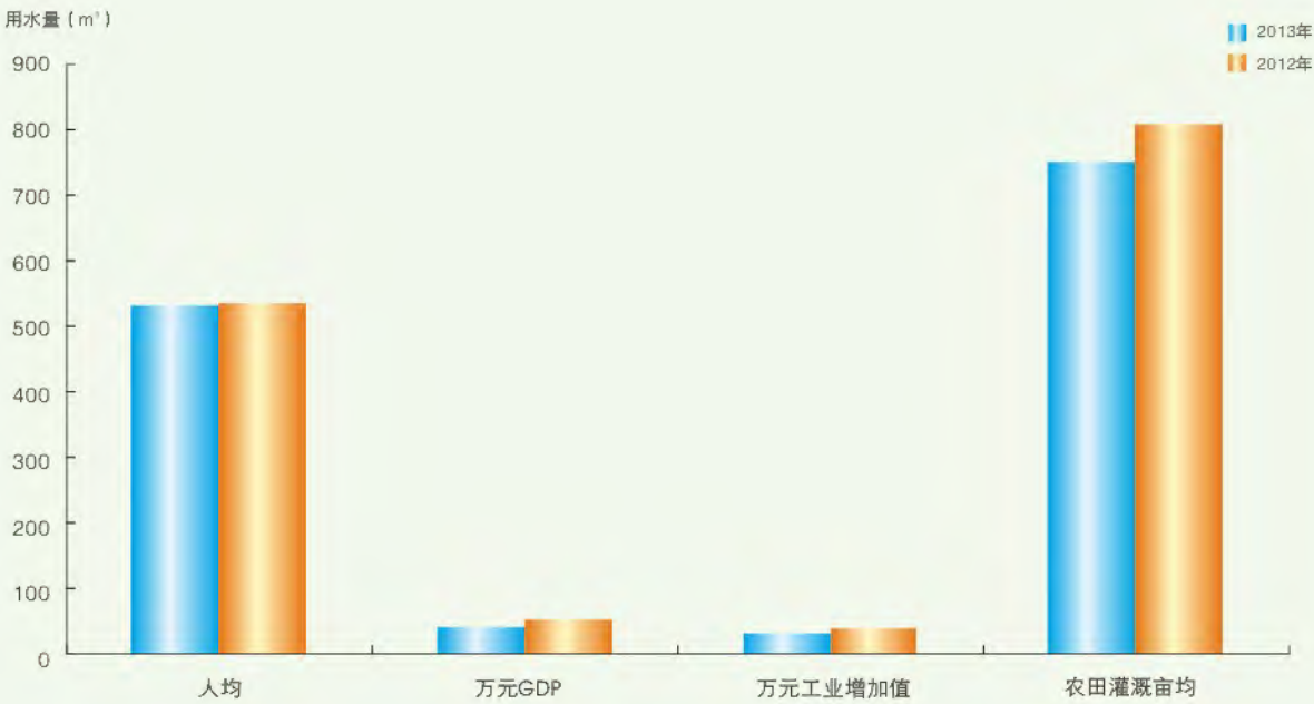
2013年与2012年各项主要用水指标比较图
