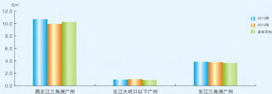
各水资源分区2013年地下水资源量与2012年、多年平均比较图
