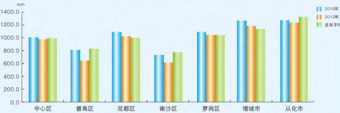
各行政区2013年地表径流深与2012年、多年平均比较图
