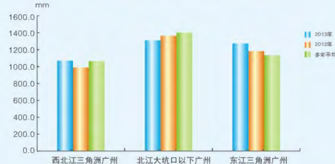
各水资源分区2013年径流深与2012年、多年平均比较图
