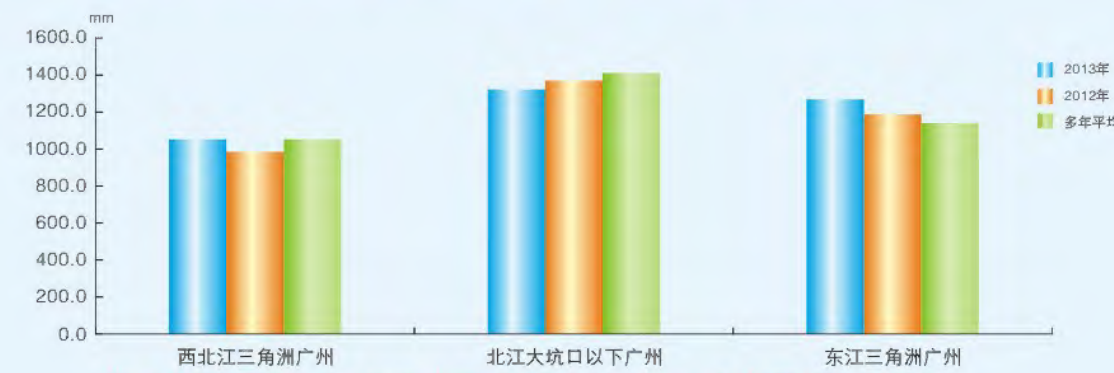
各水资源分区2013年地表径流深与2012年、多年平均比较图
