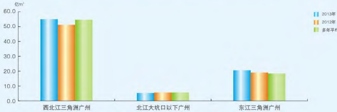
各水资源分区2013年地表水资源量与2012年、多年平均比较图
