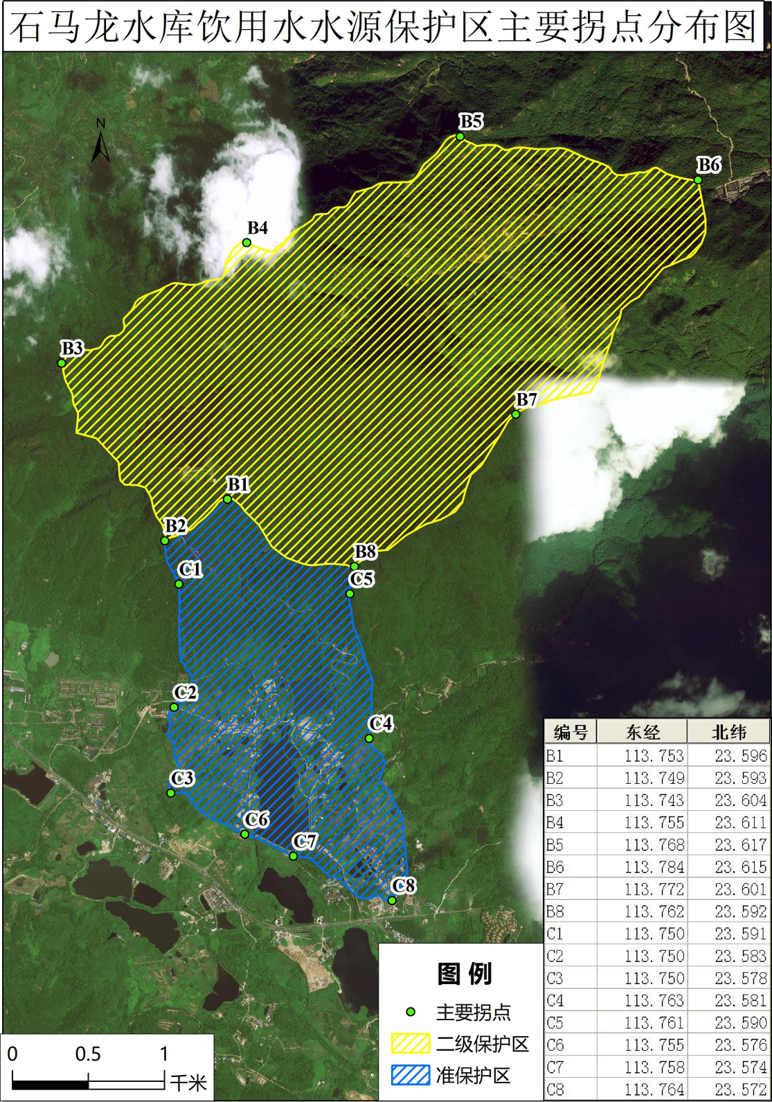
石马龙水库饮用水水源保护区主要拐点分布图及坐标
