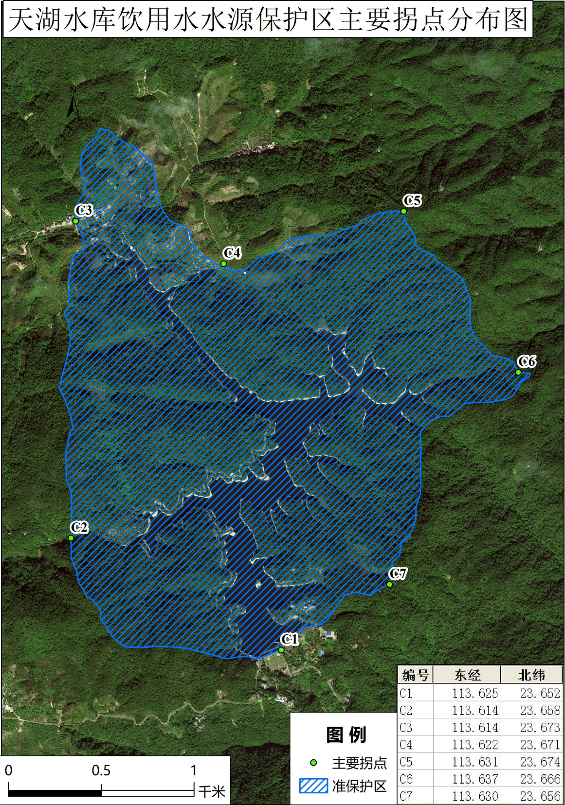
天湖水库饮用水水源保护区主要拐点分布图及坐标
