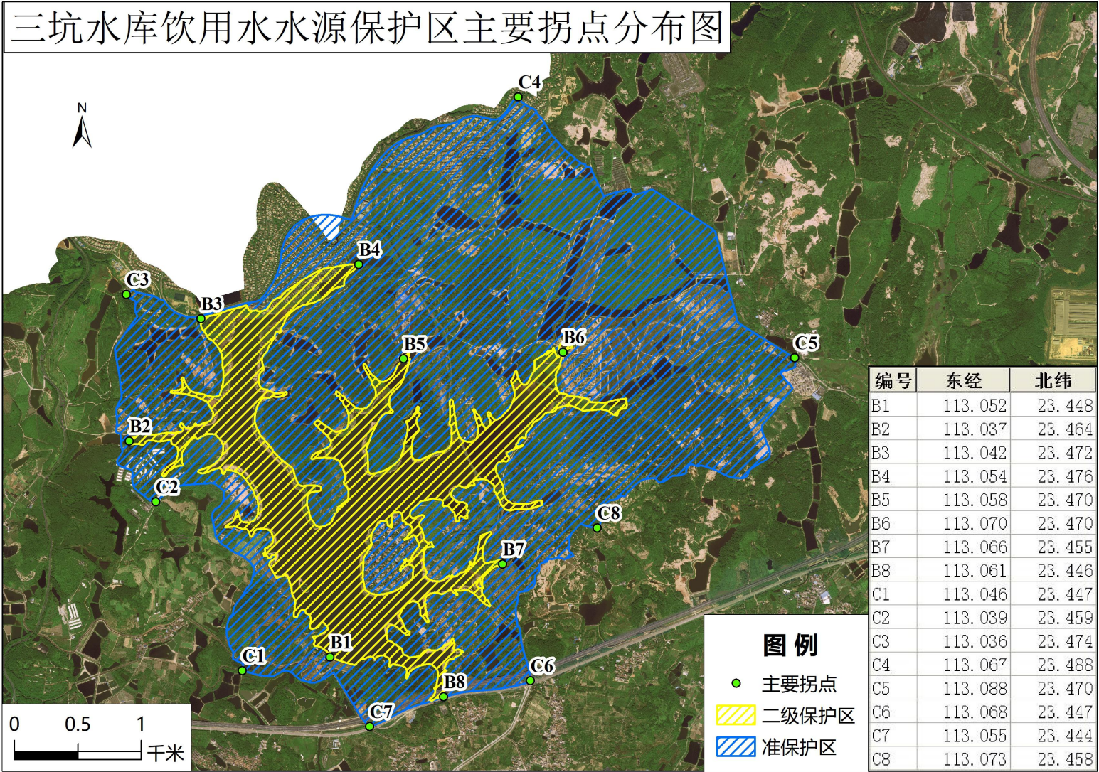
三坑水库饮用水水源保护区主要拐点分布图及坐标
