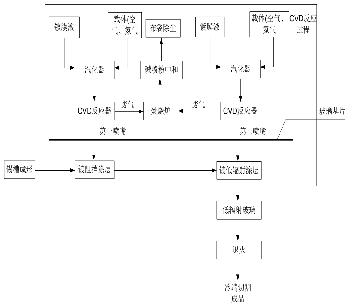
图 A.2 典型玻璃制品镀膜工序工艺流程-化学气相沉积工艺（CVD）
