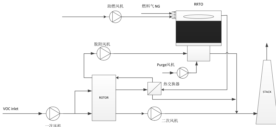
图 1 转轮吸附浓缩加蓄热燃烧工艺
