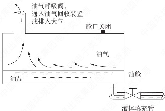
图 1-7 底部装载
