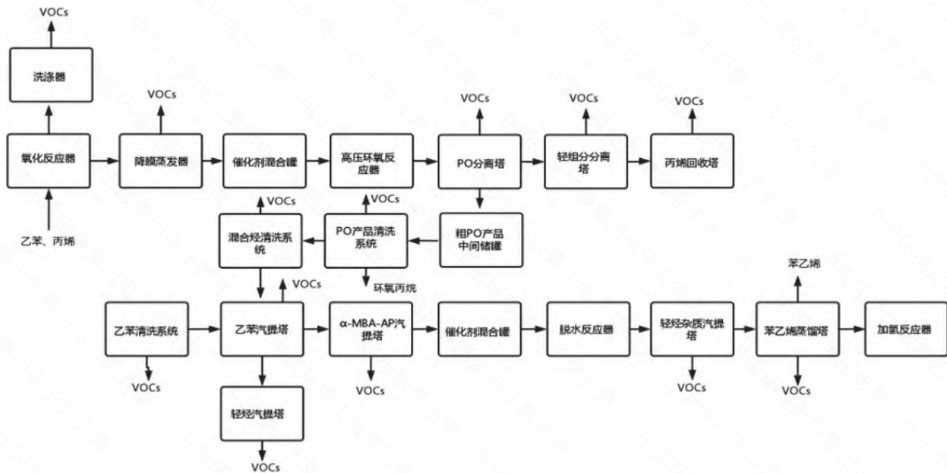
图 1-15 乙苯共氧化法制环氧丙烷 / 苯乙烯 (PO/SM) 生产工艺流程与 VOCs 排放环节示意
