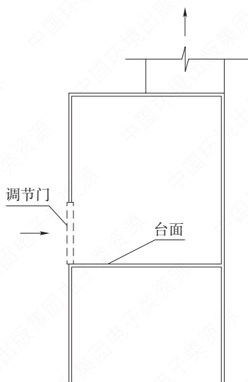
图 3-11 半密闭罩
