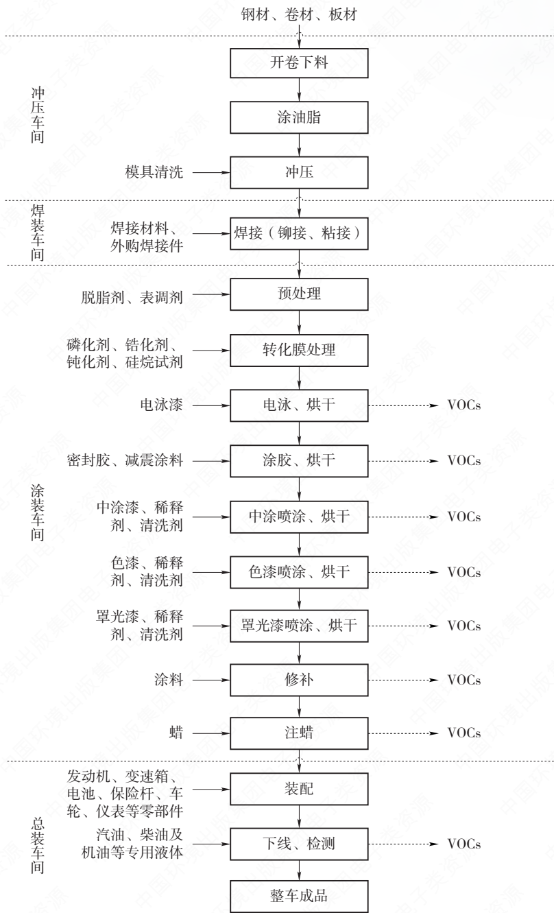
图 1-48 汽车整车制造生产工艺流程与 VOCs 排放环节示意
