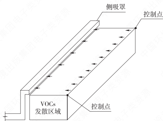
图 3-8 侧吸罩控制点示意
