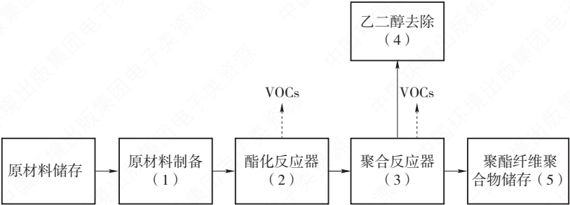
图 1-30 PET/PTA 工艺流程与 VOCs 排放环节示意
