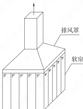
图 3-20 软帘示意
