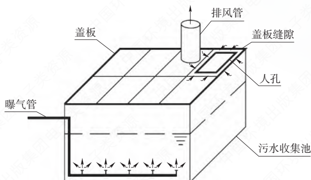
图 3-10 废水收集池密闭罩示意图
