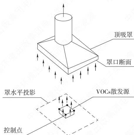
图 3-7 顶吸罩控制点示意
