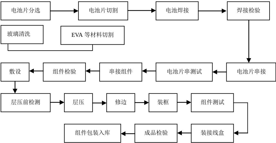
图 A. 2 太阳能电池组件主要工艺流程
