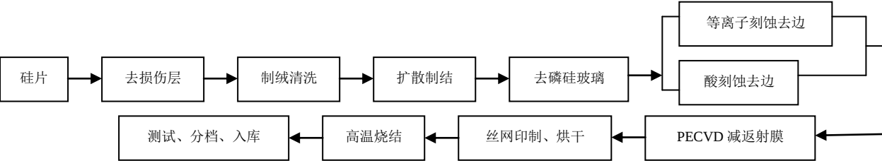
图 A. 1 硅太阳能电池片主要生产工艺流程
