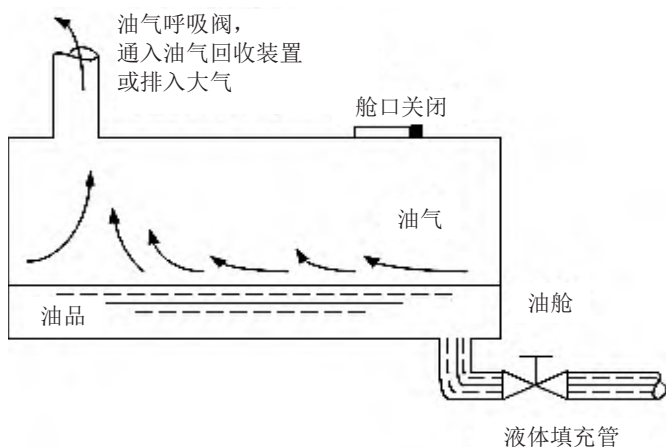
图 1-6 底部装载
