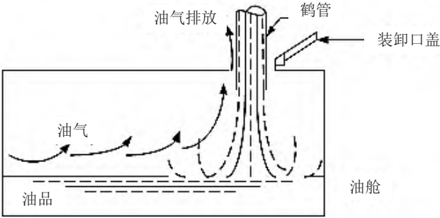
图 1-4 喷溅式装载
