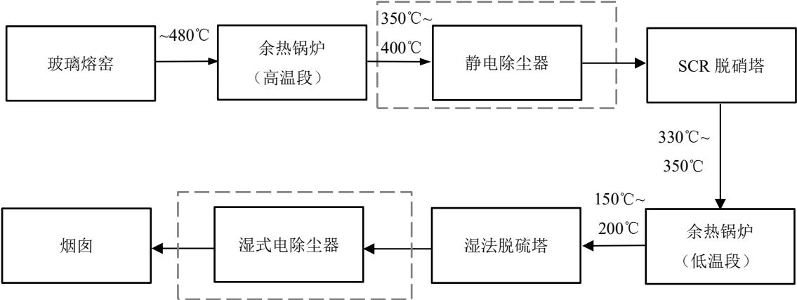
a) 静电除尘+SCR 脱硝+湿式脱硫+湿式电除尘工艺流程图
