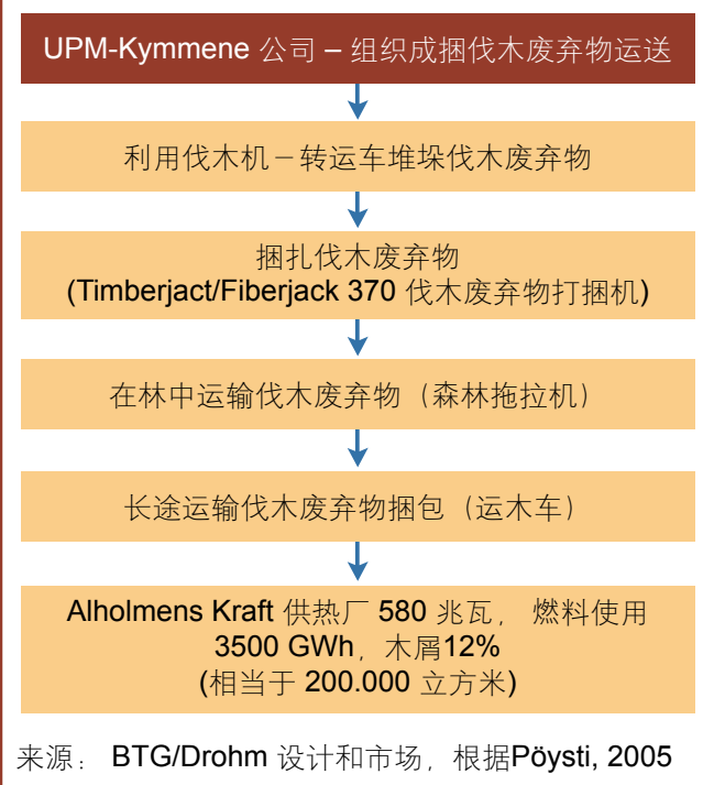
图 5.11 成捆伐木废弃物运送为基础的林业废弃物供应系统
