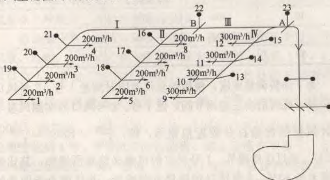
图 35 送风系统图
