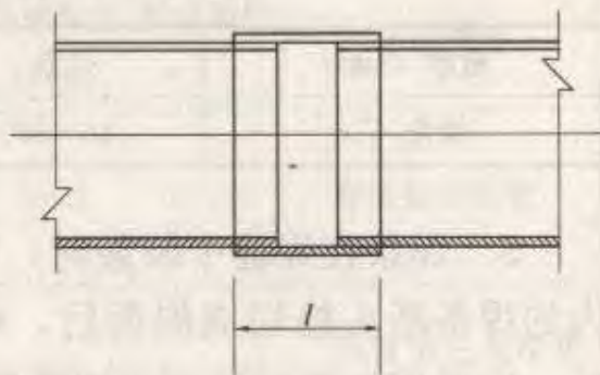
图 5.5.7-2 软接头示意
