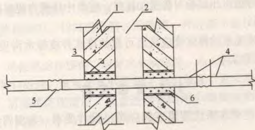
图 11.1.4-2 水管过结构变形缝墙体安装示意
