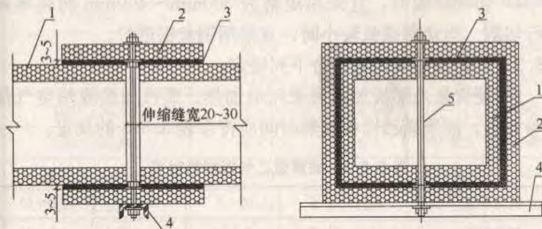
(b) 伸缩节中间设支撑柱
