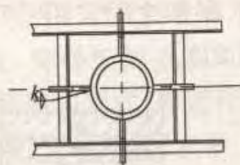
图 16 穿楼板管道
