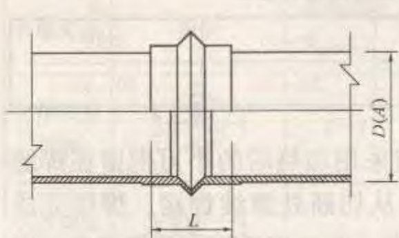
图 5.5.7-1 伸缩节示意
