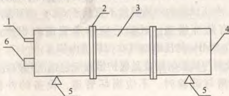
图15.2.2 漏风量测试装置连接示意
