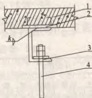
图 7 吊架与预埋件焊接固定示意
