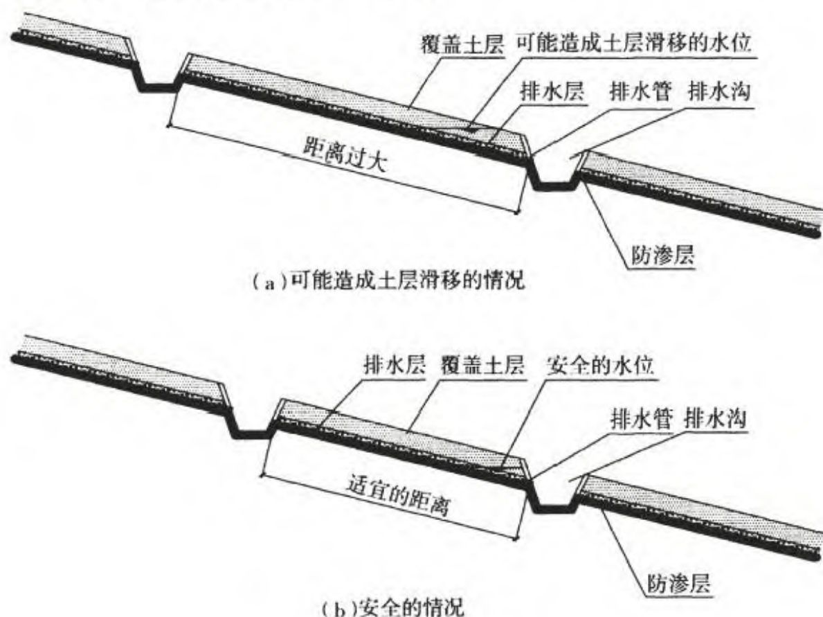
图 3 覆盖土层排水示意图
