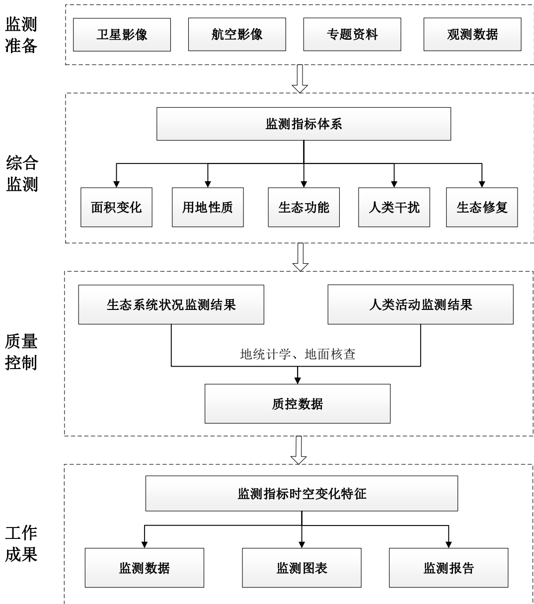
图 1 生态保护红线生态状况监测技术流程图
