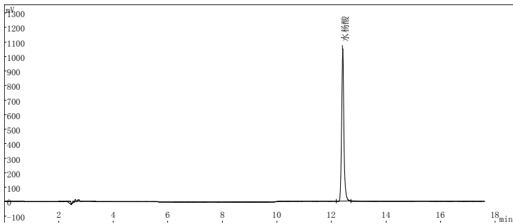
图 1 标准溶液色谱图
