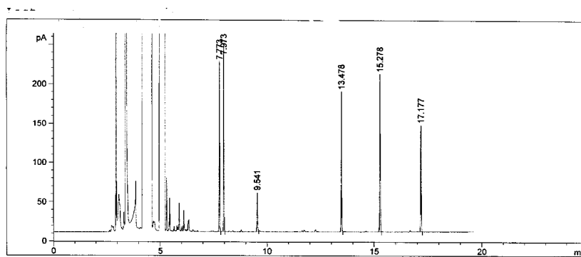
图3 标准溶液色谱图
