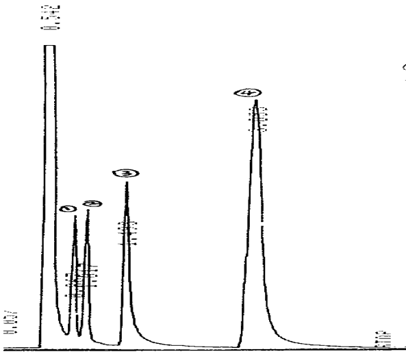
图 2 标准溶液色谱图 1: 苯酚; 3: 氢醌。
