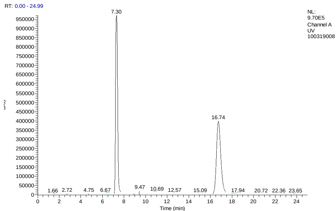
图 2 标准溶液衍生化反应后的色谱图 甲醛衍生物 (2, 4-二硝基苯腙) (16.74 min)
