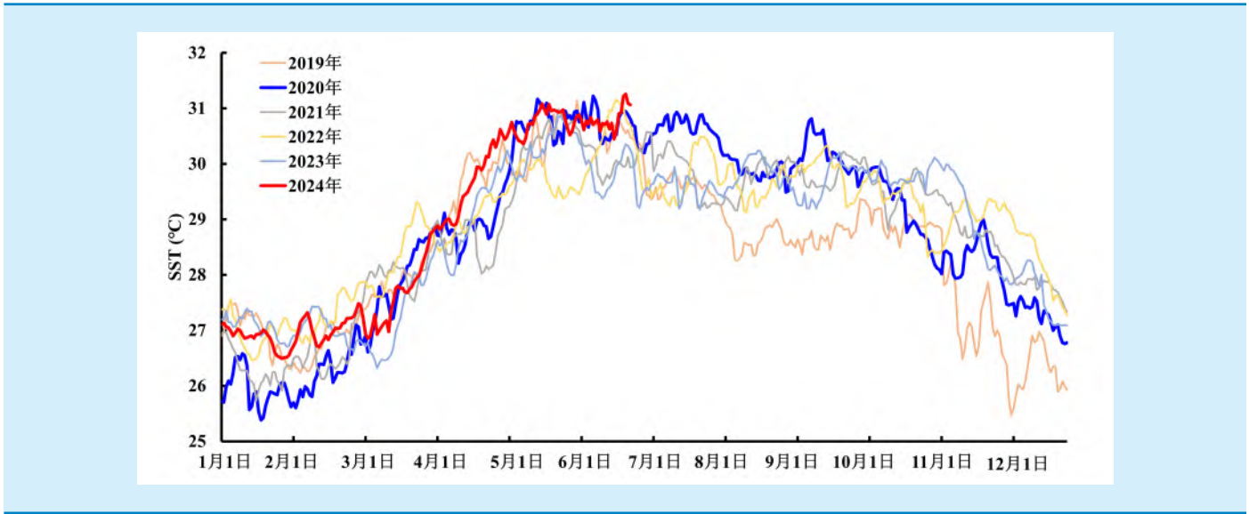
黄岩岛海域 SST 的日际变化对比（2019 年~2024 年）
