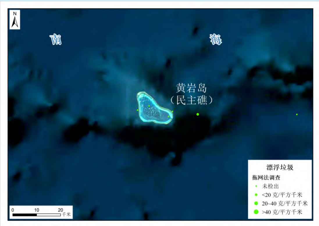
黄岩岛海域漂浮垃圾分布示意图（2024 年 5 月 ~6 月，拖网法）
