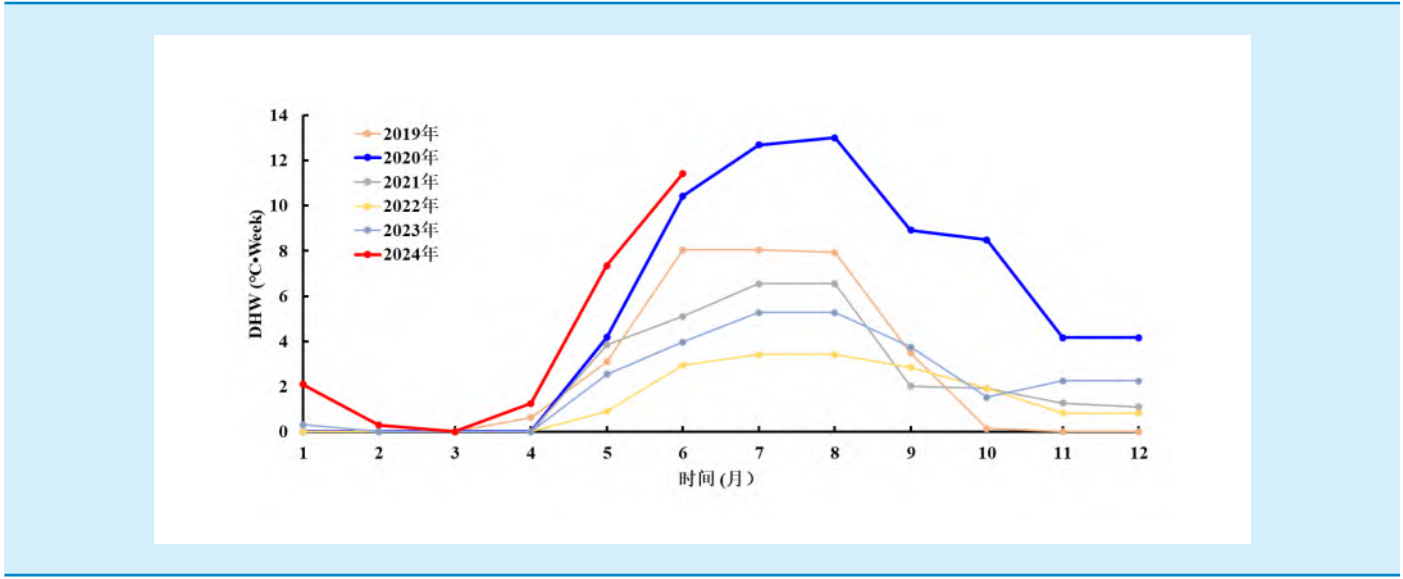
黄岩岛海域 DHW 的月际变化对比（2019 年~2024 年）
