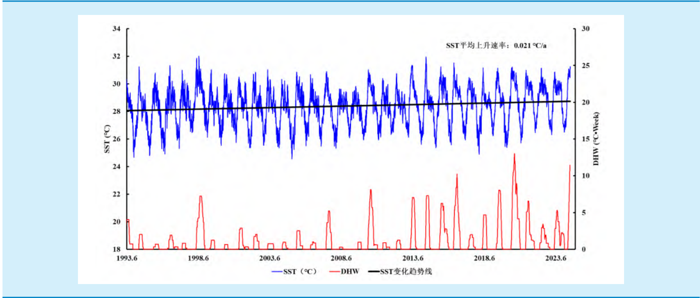
黄岩岛海域 SST 和 DHW 的时间变化曲线（1993 年~2024 年）
