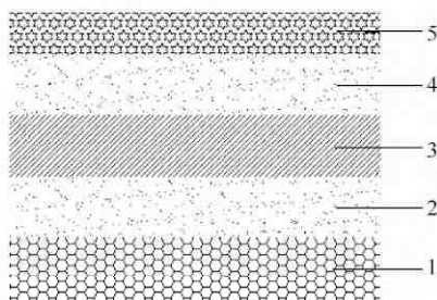
图 10.8.4 封场覆盖系统示意
