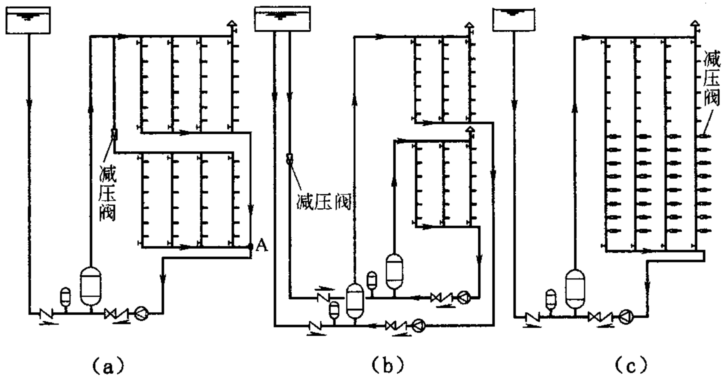
图3 减压阀设置
