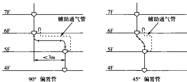
(d) 偏置管设置辅助通气管模式
