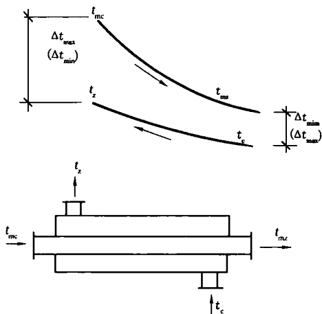
图6 快速水加热器水加热工况示意
