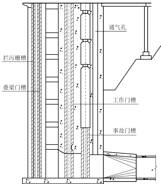
(a) 事故闸门在边坡外
