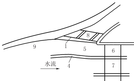
(b) 布置形式二
