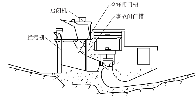
图 3 河床式进水口
