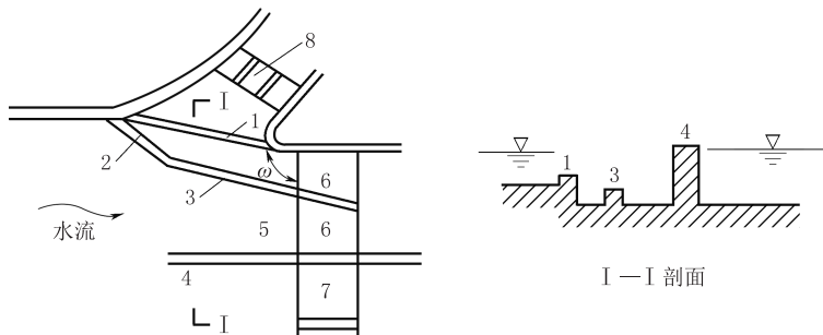
(a) 布置形式一
