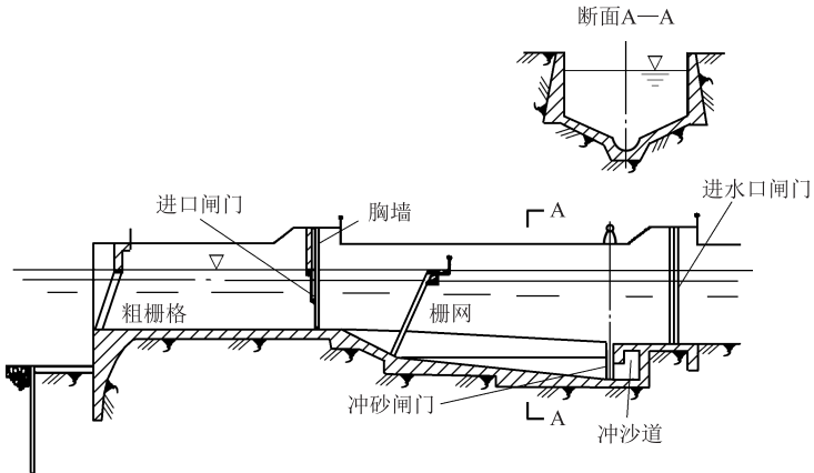
图 13 拦河闸式进水口
