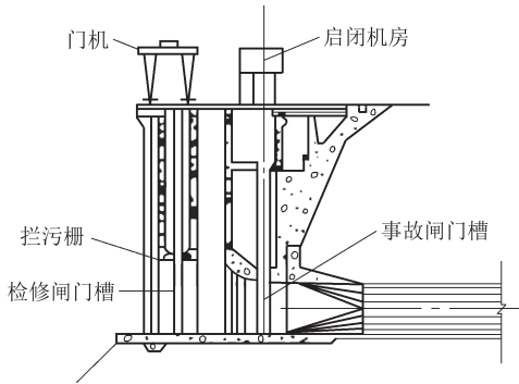
图 4 岸塔式进水口
