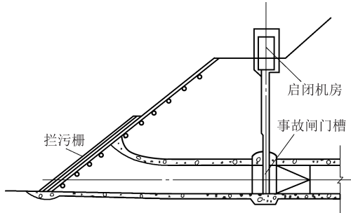
图 6 竖井式进水口
