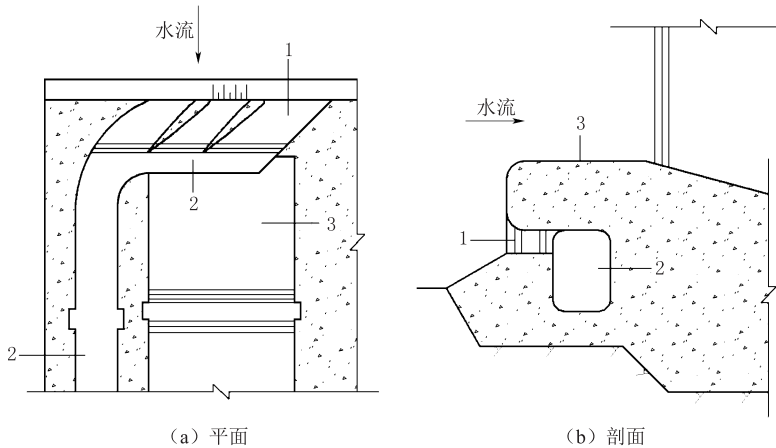
图 C.5.2-3 河床式水电站厂房墩内排沙管（或排沙廊道）进水口
