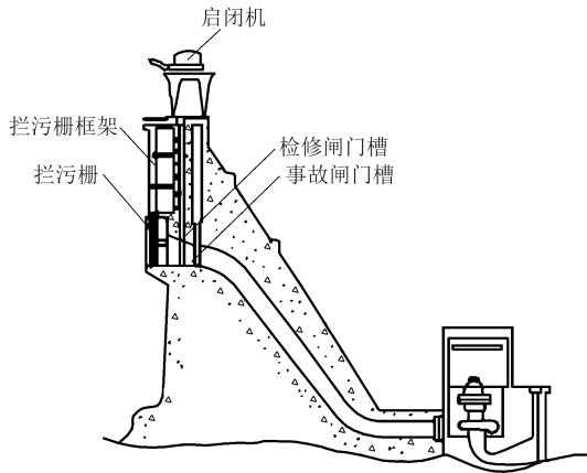
图 1 坝式进水口
