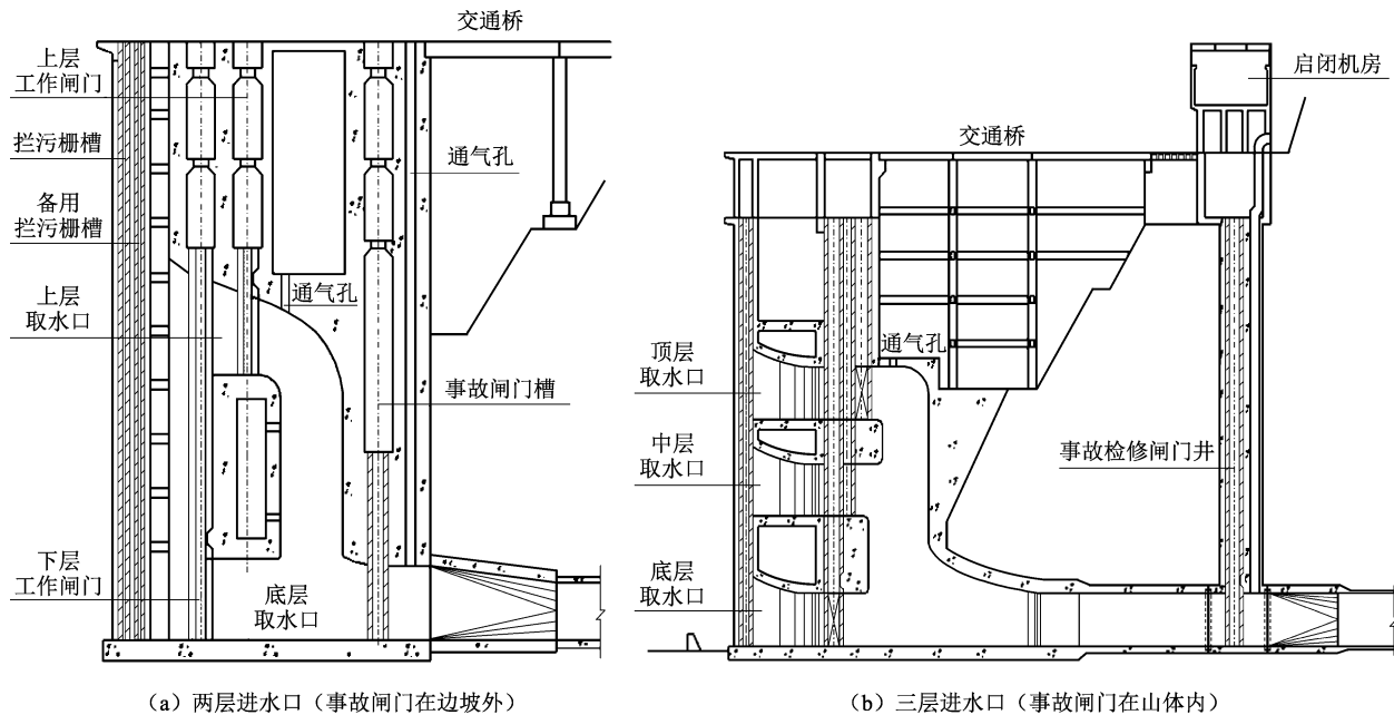
图 11 多层进水口
