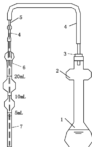
1—100 mL 容积发生瓶；2—硼氢化钾存放处；3—橡皮塞；4—乳胶软管； 5—塑料管（一端拉成毛细管状，出气口内径小于 1 mm）；6—14 mm 标准磨口；7—吸收液，高度不低于 5 cm
