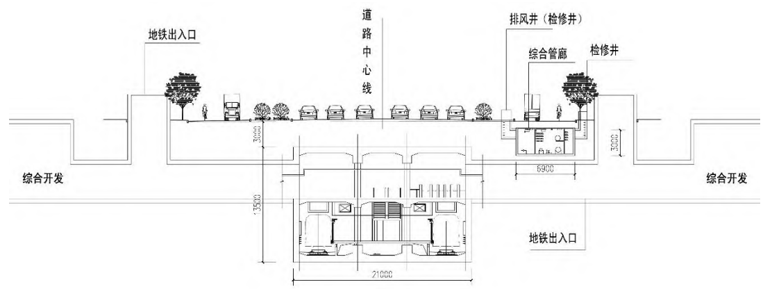
图7.26 综合管廊与轨道同步建设位置关系图
