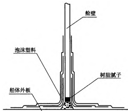
图 A.4.1 (1) 单板舱壁与船体外板的连接
