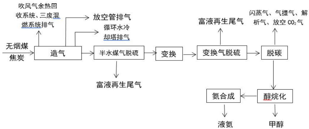
图 25-4 固定床常压间歇煤气化工艺合成氨生产工艺流程图
