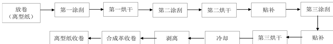
图 33-4 聚氨酯干法工艺生产工艺流程图
