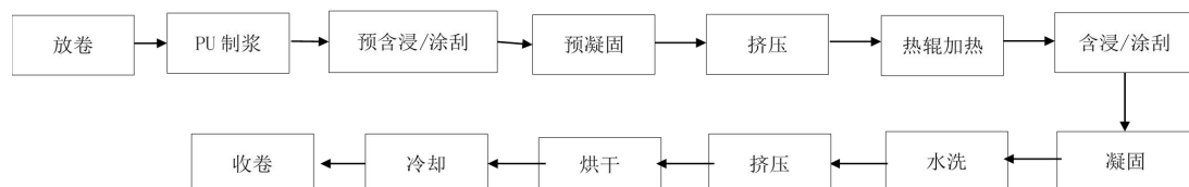
图 33-5 聚氨酯湿法工艺生产工艺流程图
