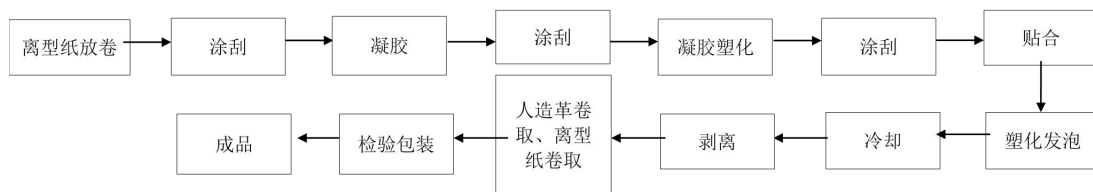
图 33-2 聚氯乙烯离型纸法生产工艺流程图
