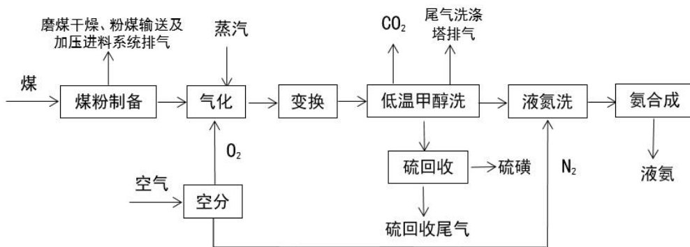
图 25-2 干煤粉气流床气化工工艺合成氨生产工艺流程图
