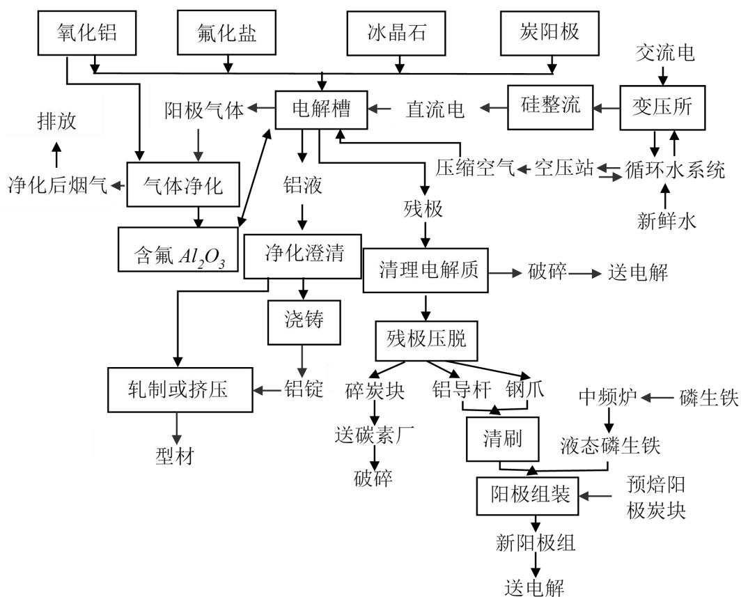
图 8-1 电解铝生产工艺流程图
