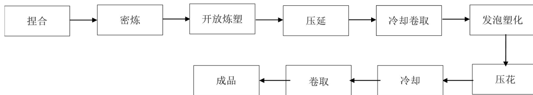
图 33-3 聚氯乙烯压延法生产工艺流程图
